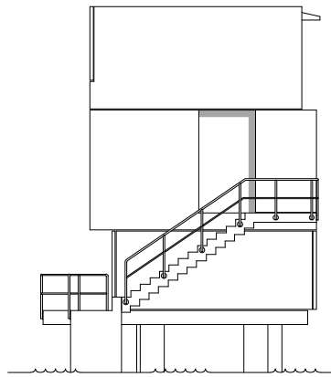
Süd-Fassade 0 1 2 [m]
