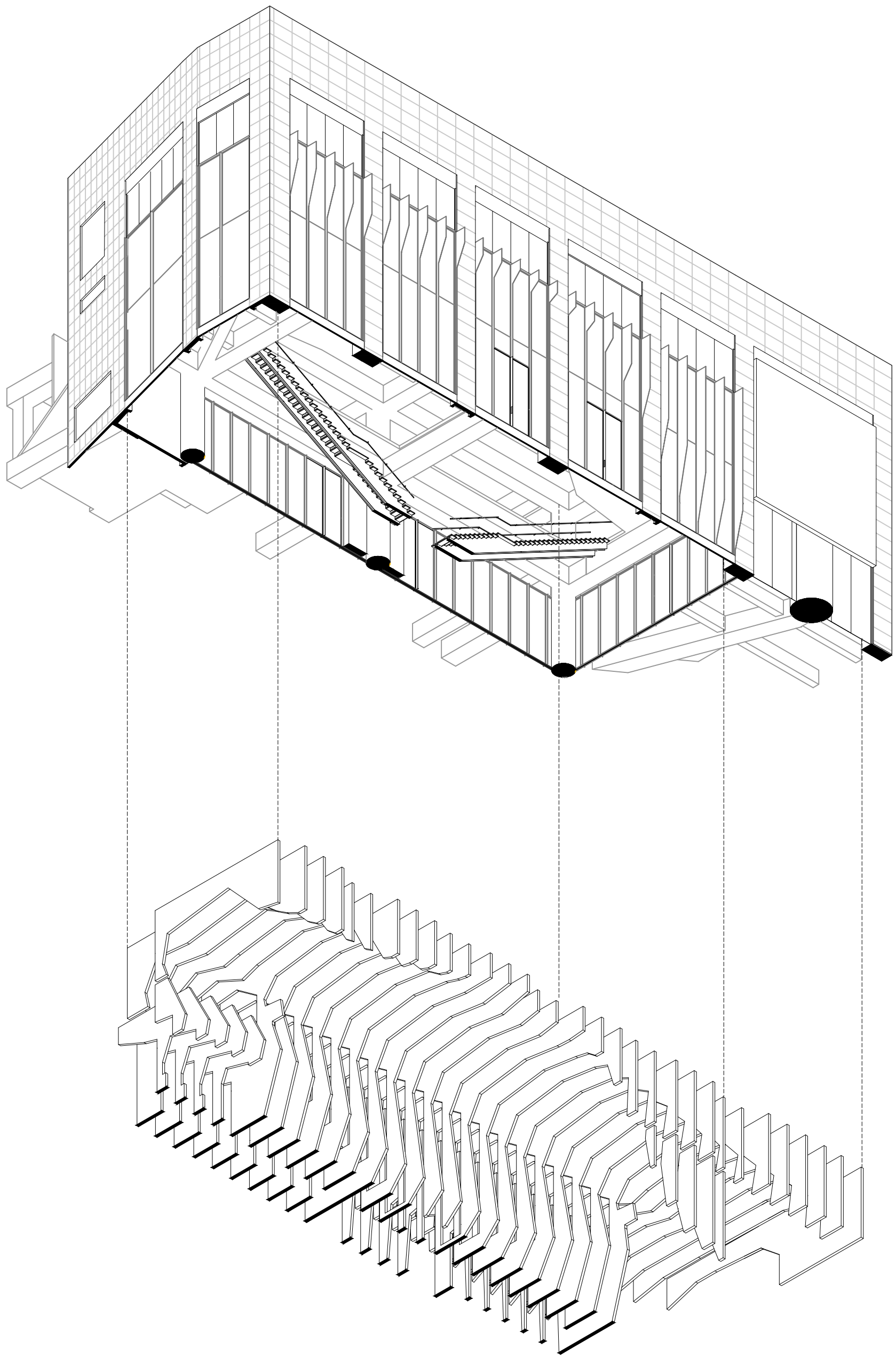
AXONOMETRIC
