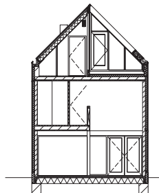
Dwarsdoorsnede
