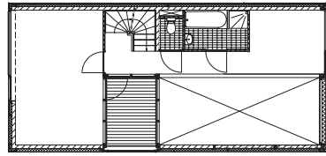
1e verdieping
