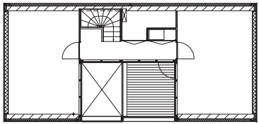
2e verdieping
