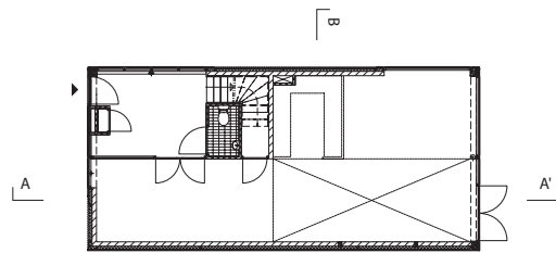
Begane grond
