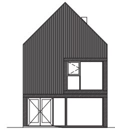
Kopgevel
