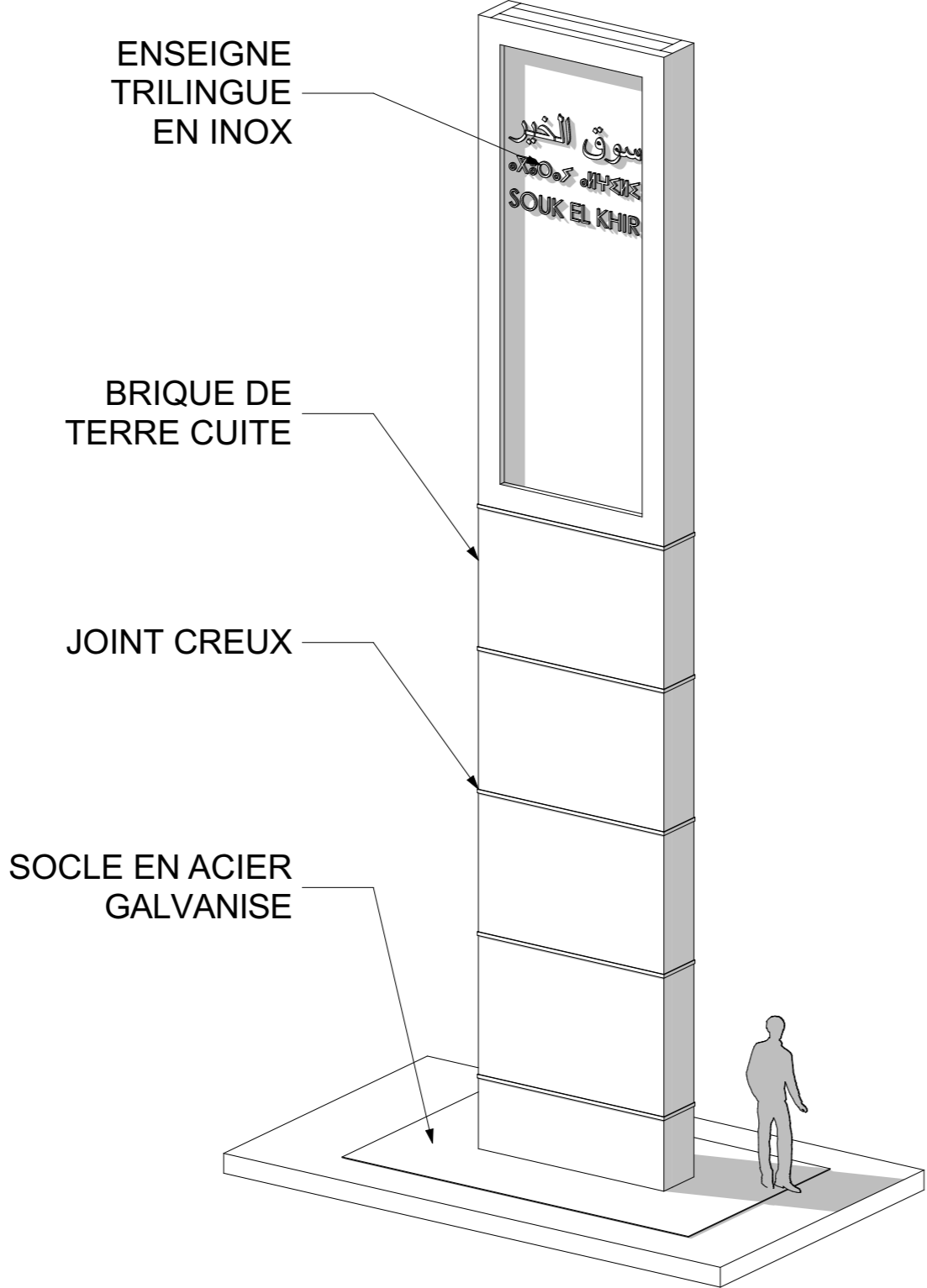
AXONOMETRIE TOTEM
