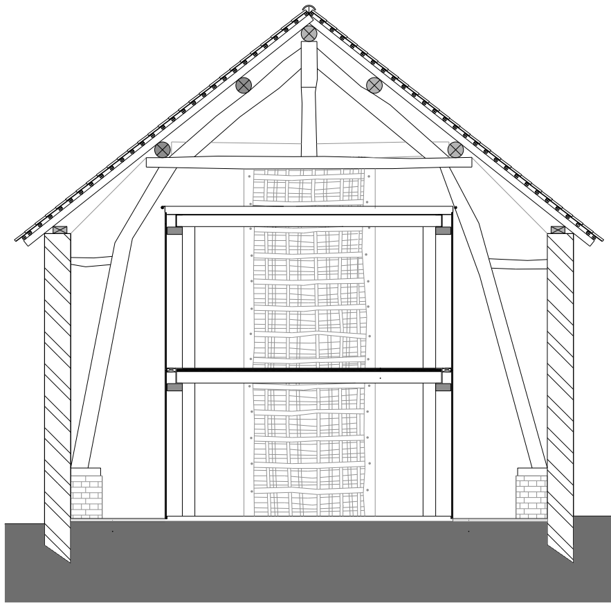
Doorsnede BB'
