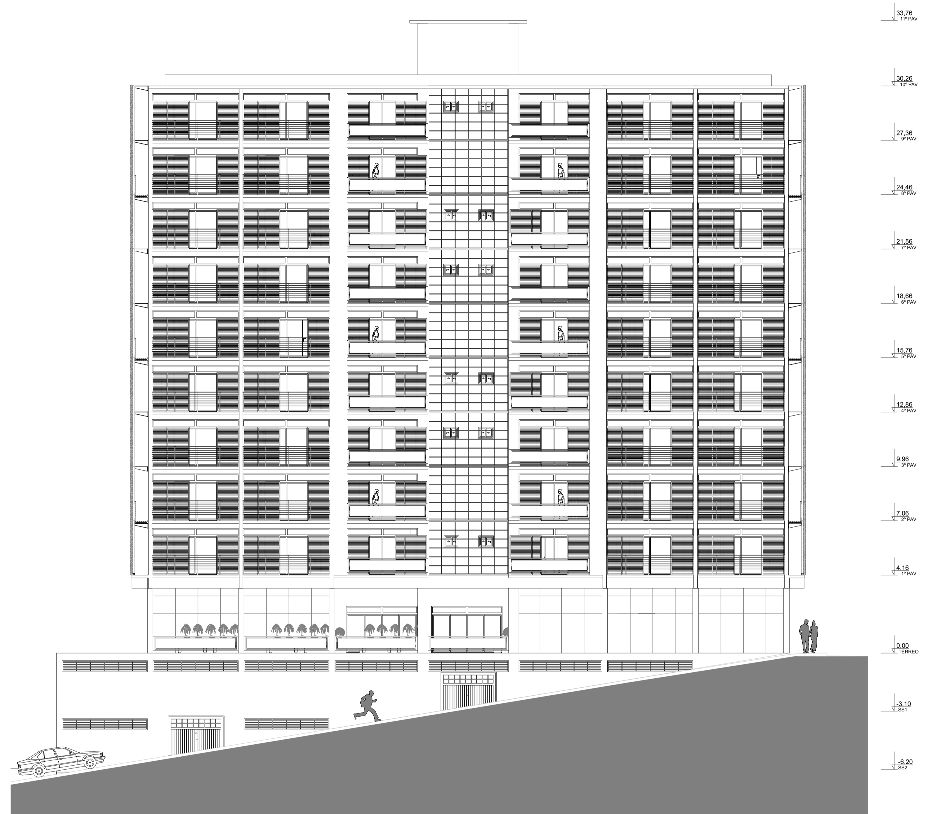
FACHADA LESTE
