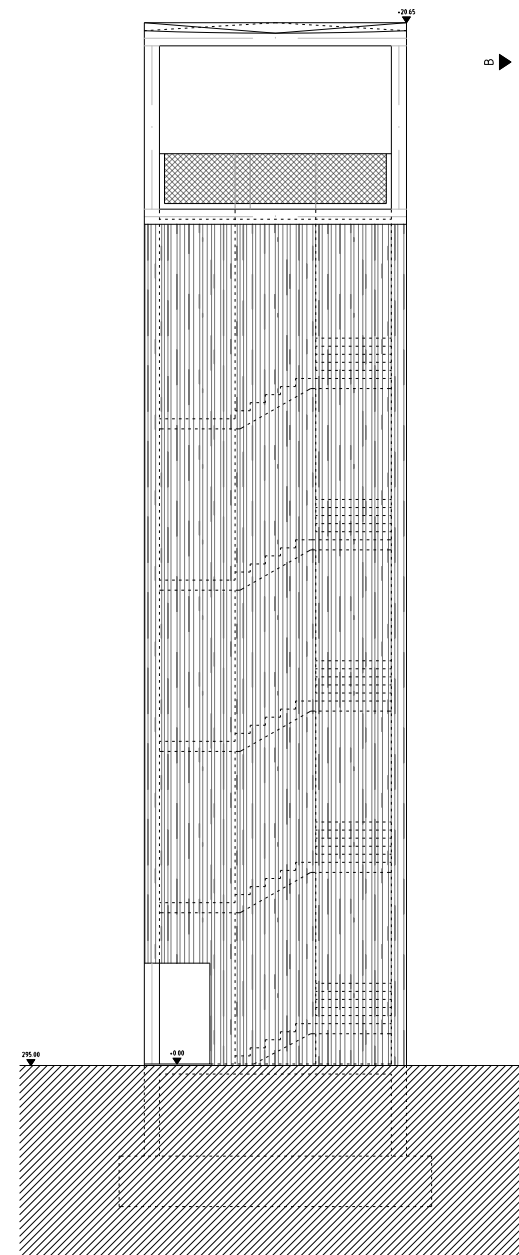
ELEVATION B
