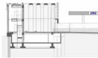
Sezione trasversale
