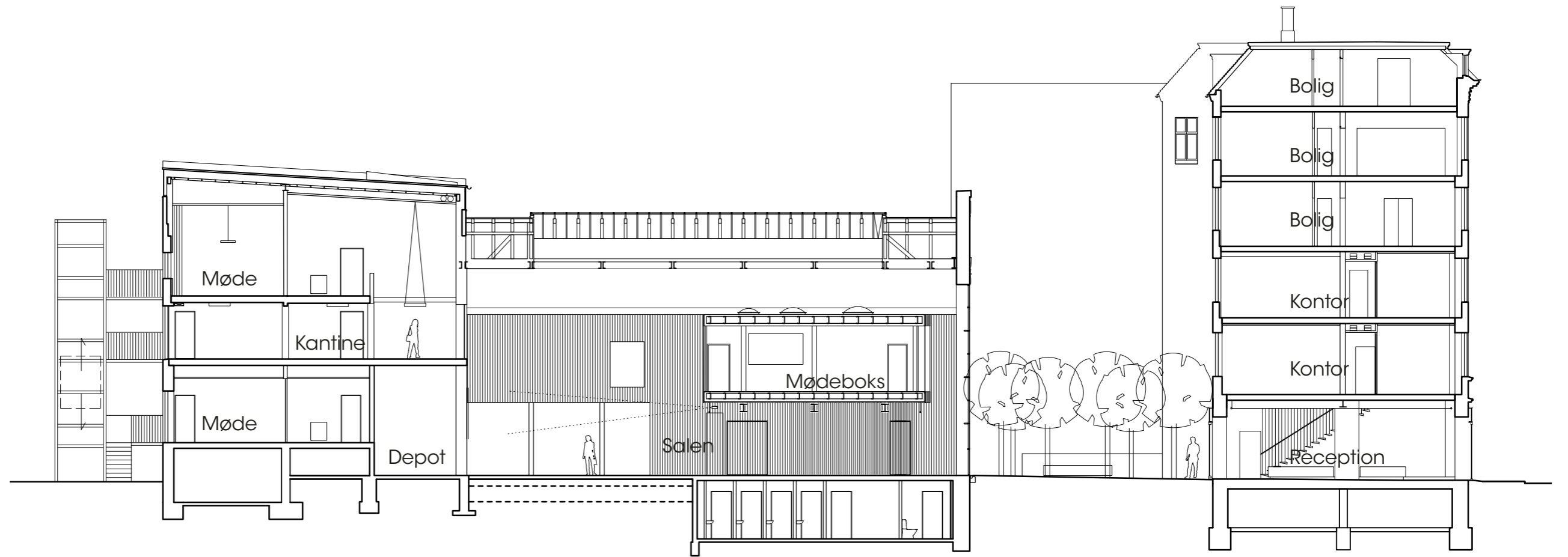
snit A-A 1:200
