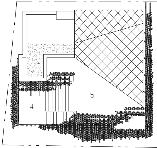
屋上平面図
