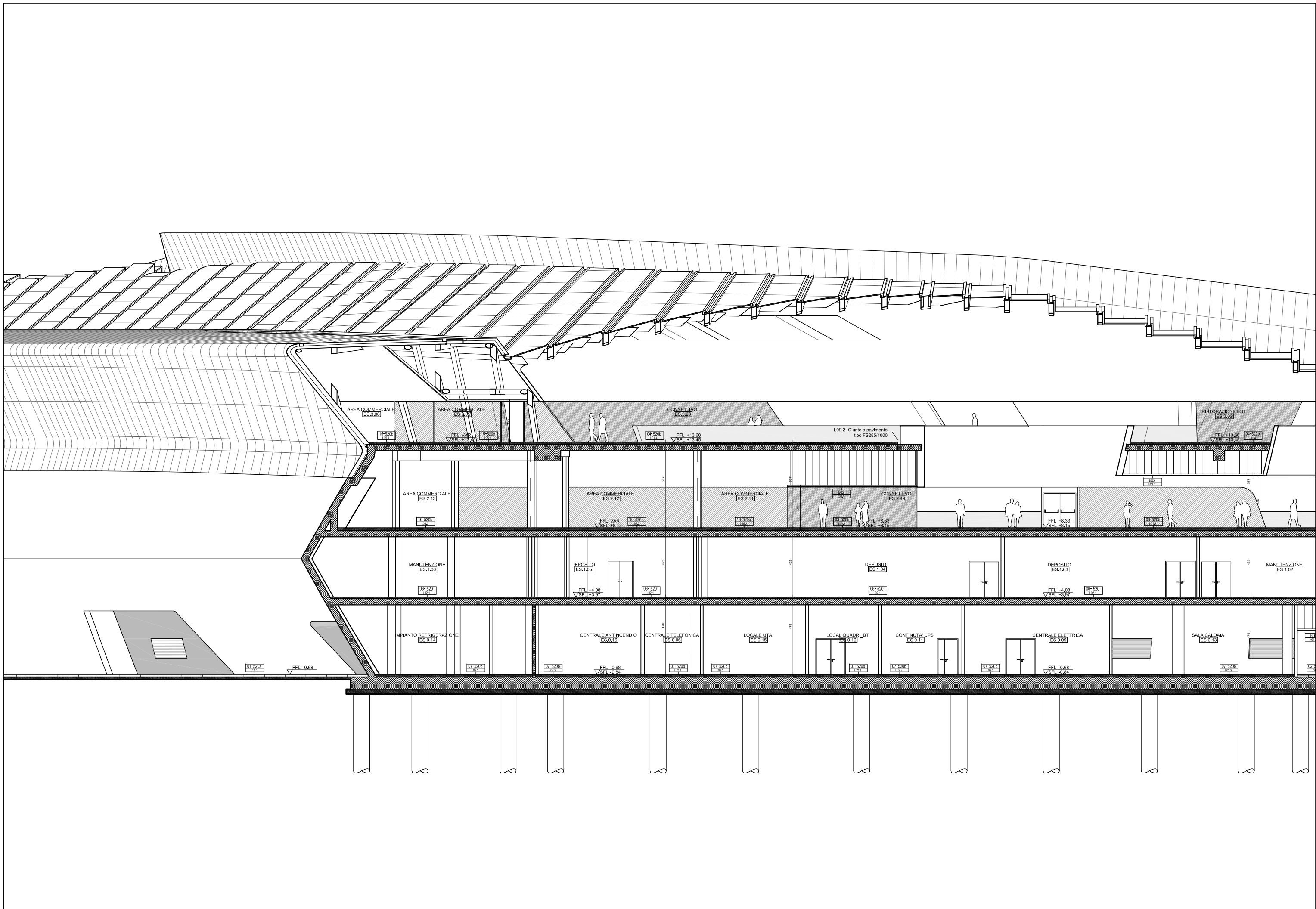
Sezione 232a
