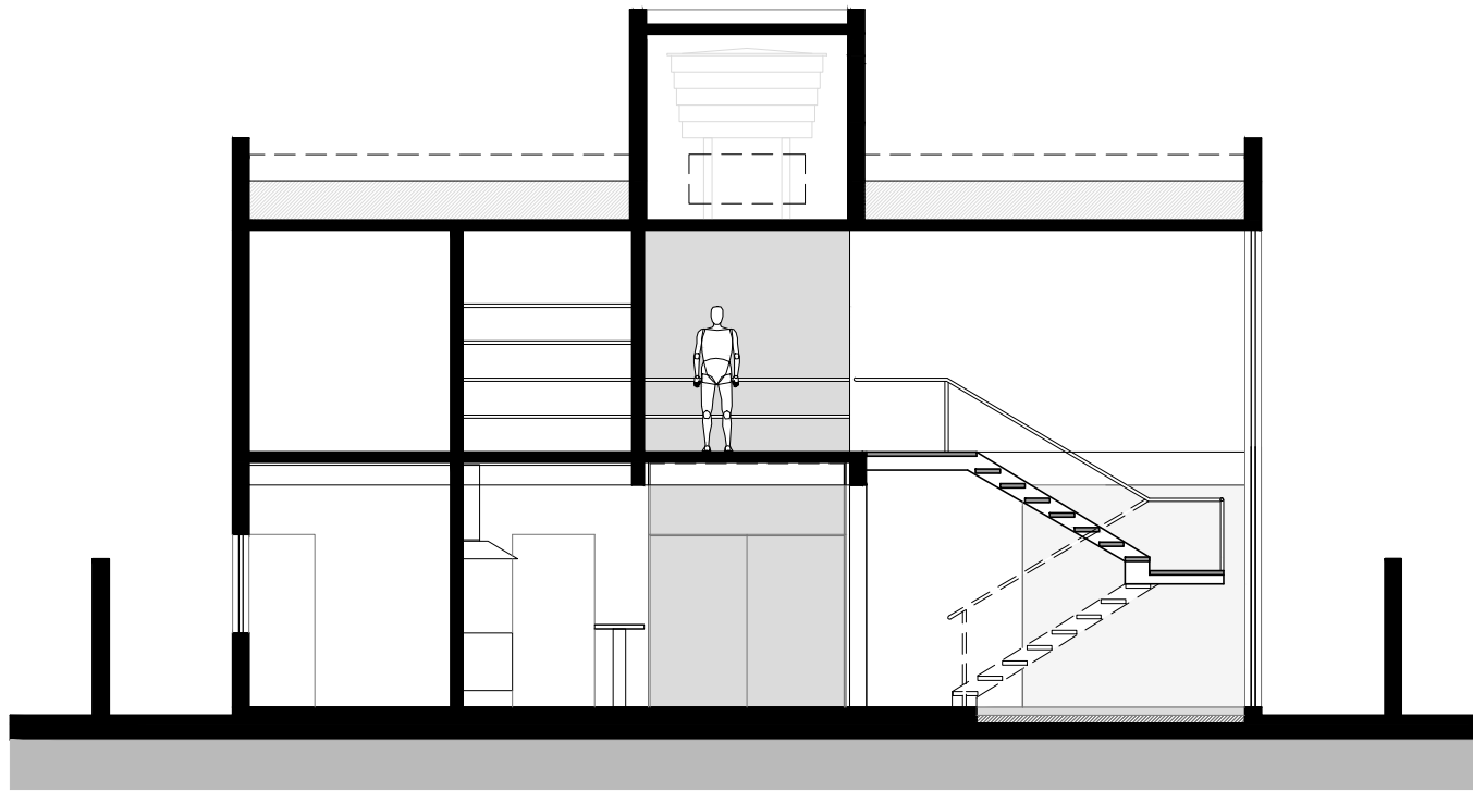
SECCIÓN AA
