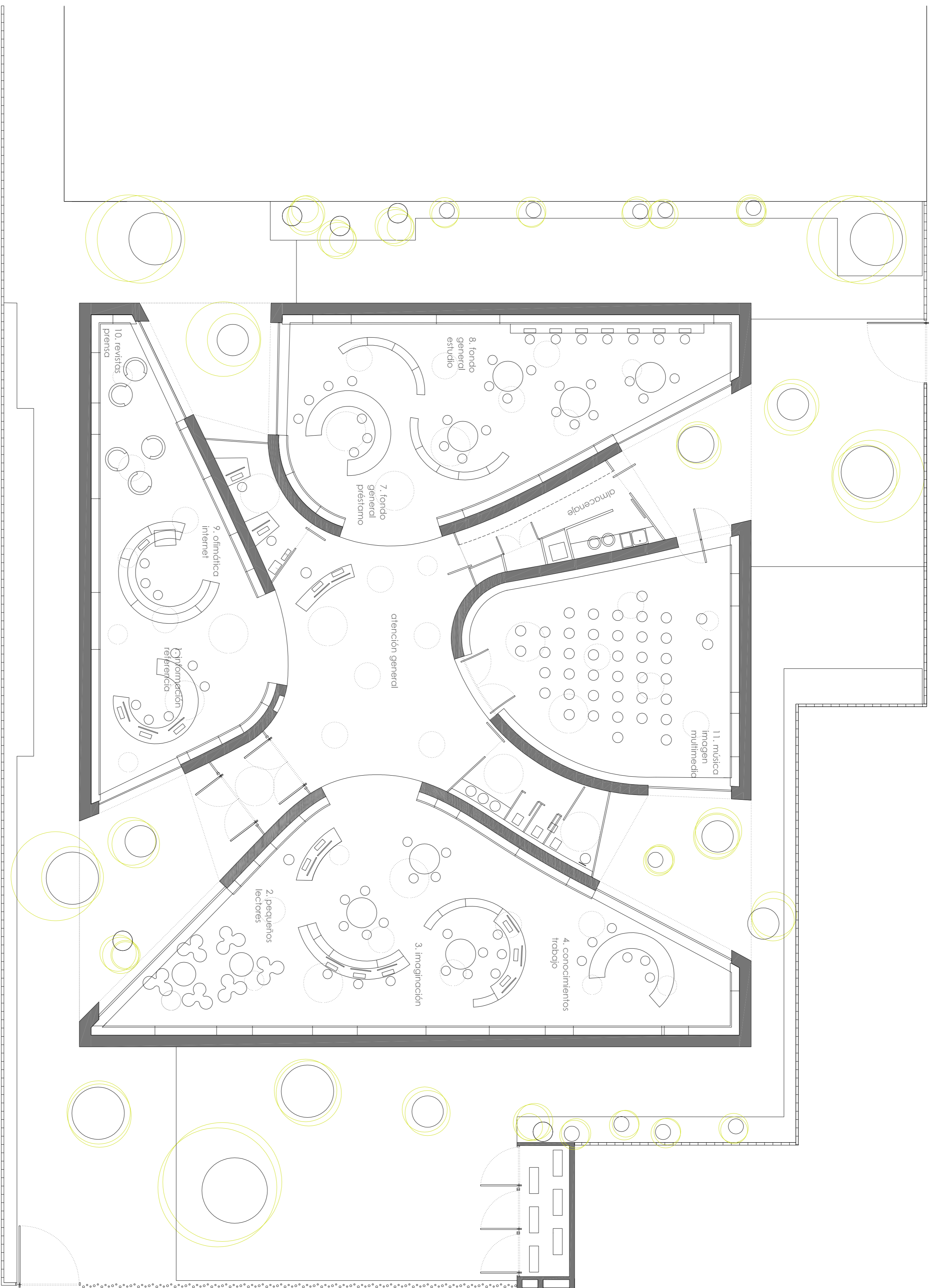
PLANTA BAJA
