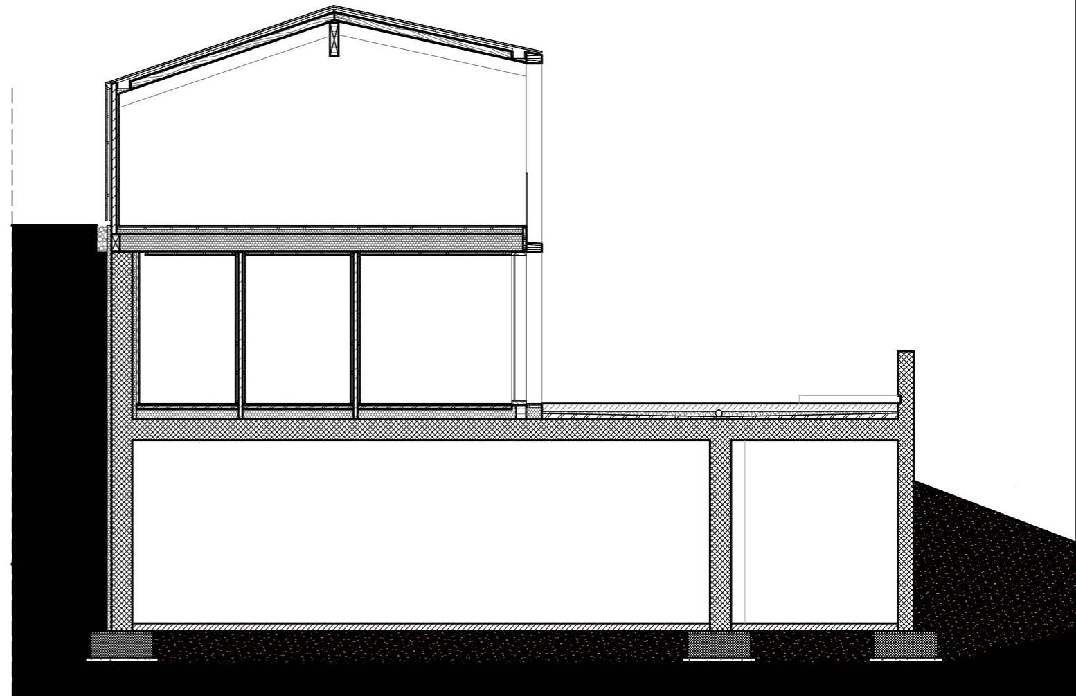
sezione bb 1:100
