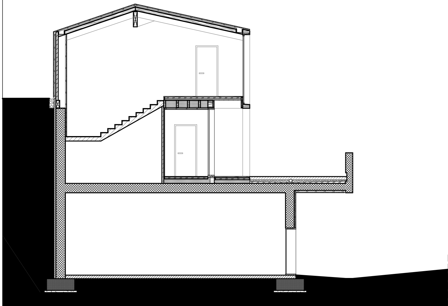
sezione aa 1:100
