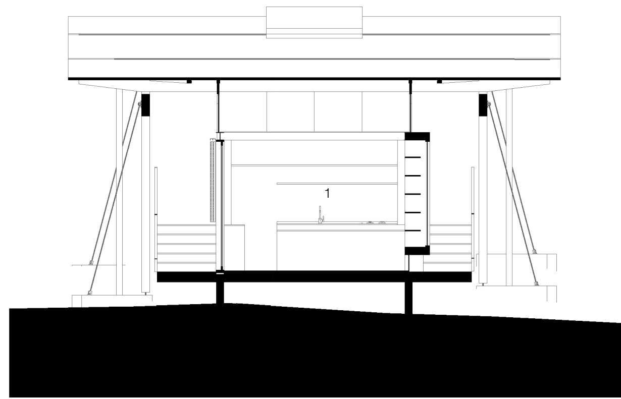
corte d 1. sala de aula
