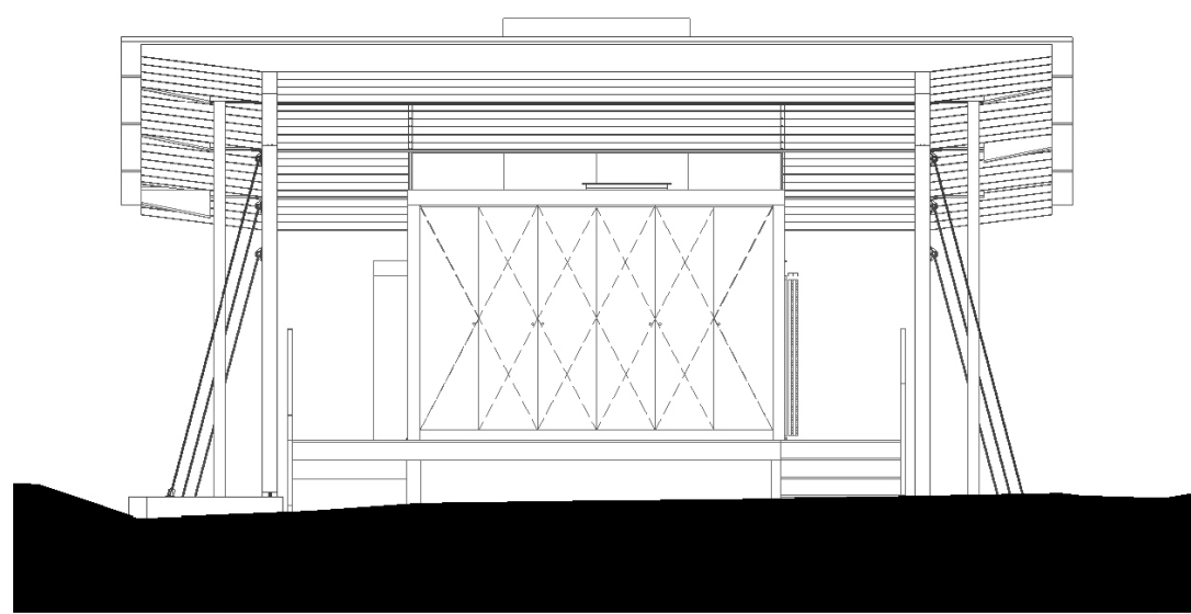
elevação sudeste
