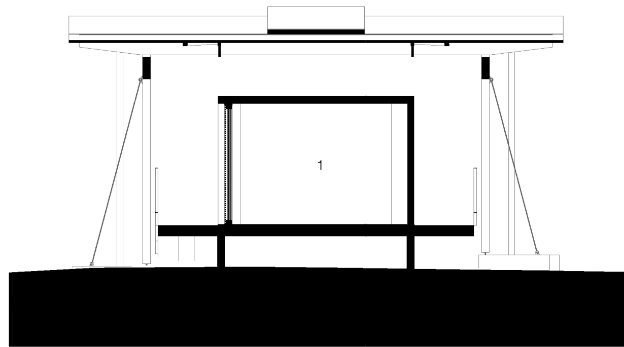
corte e 1. depósito de sementes
