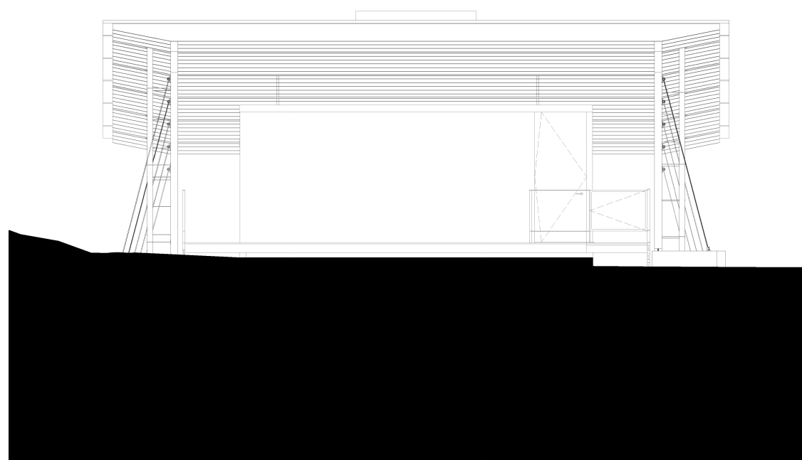
elevação sudeste
