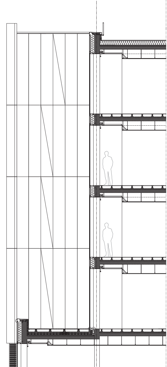
COUPE FAILLE
