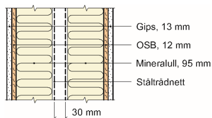
Fig. 3 Prinsipiell oppbygning av leilighetsskillevegg
