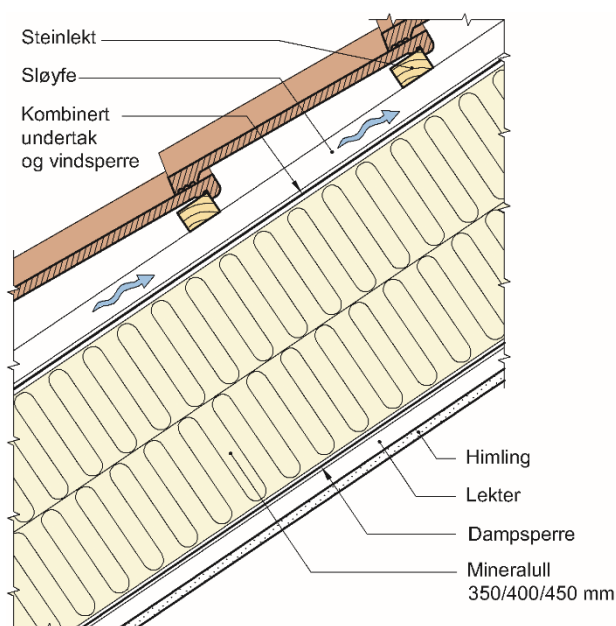
Fig. 5 Prinsipiell oppbygning av isolert takelement
