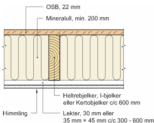
Fig. 4 Prinsipiell oppbygning av etasjeskiller innenfor samme boenhet
