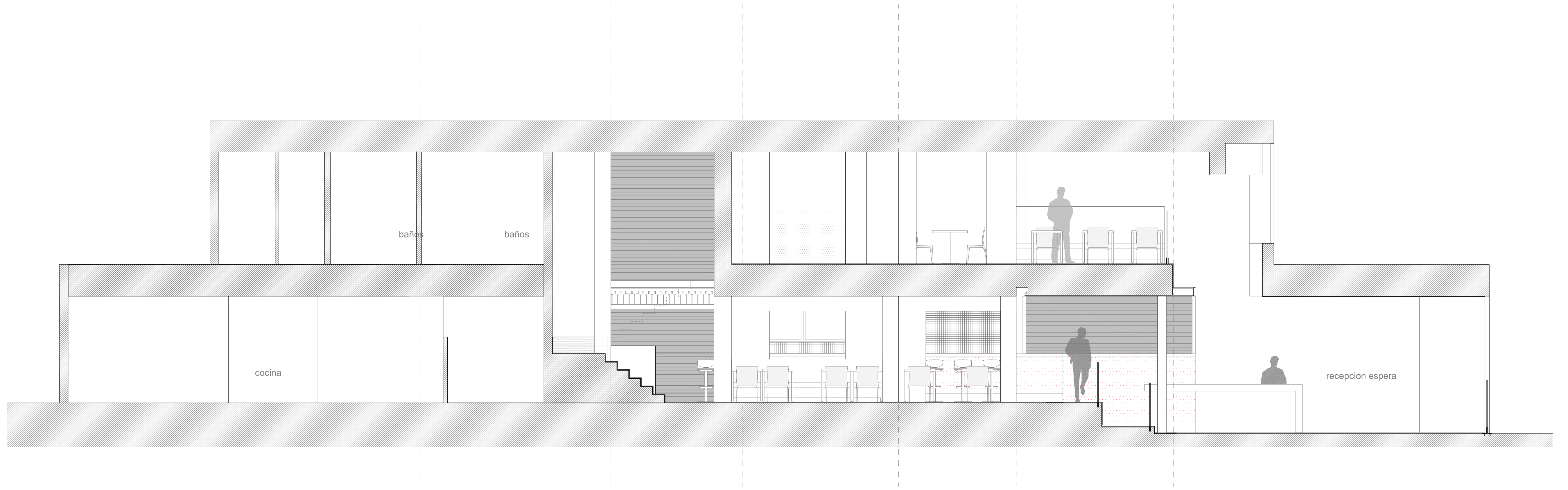
corte X2
