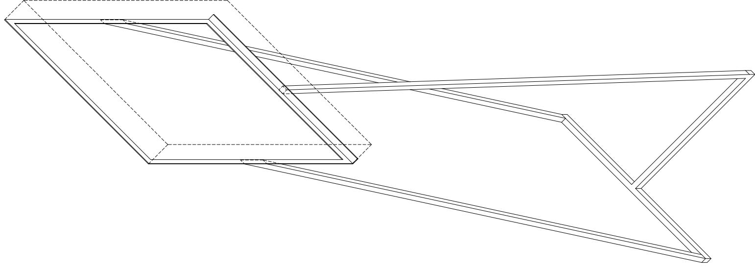
ASSONOMETRIA STRUTTURA METALLICA 1/10
