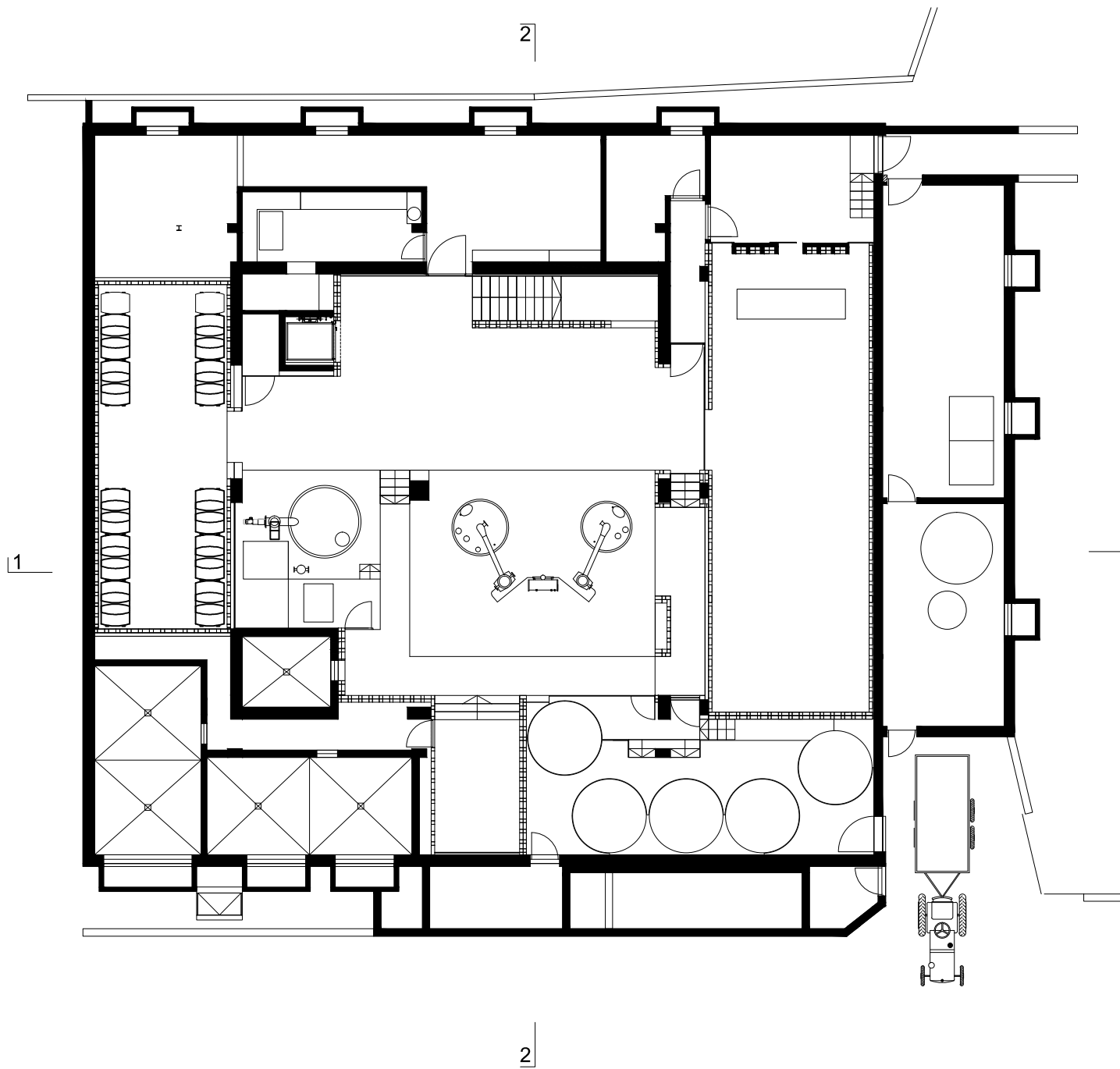
UNTERGESCHOSS -4,60m
