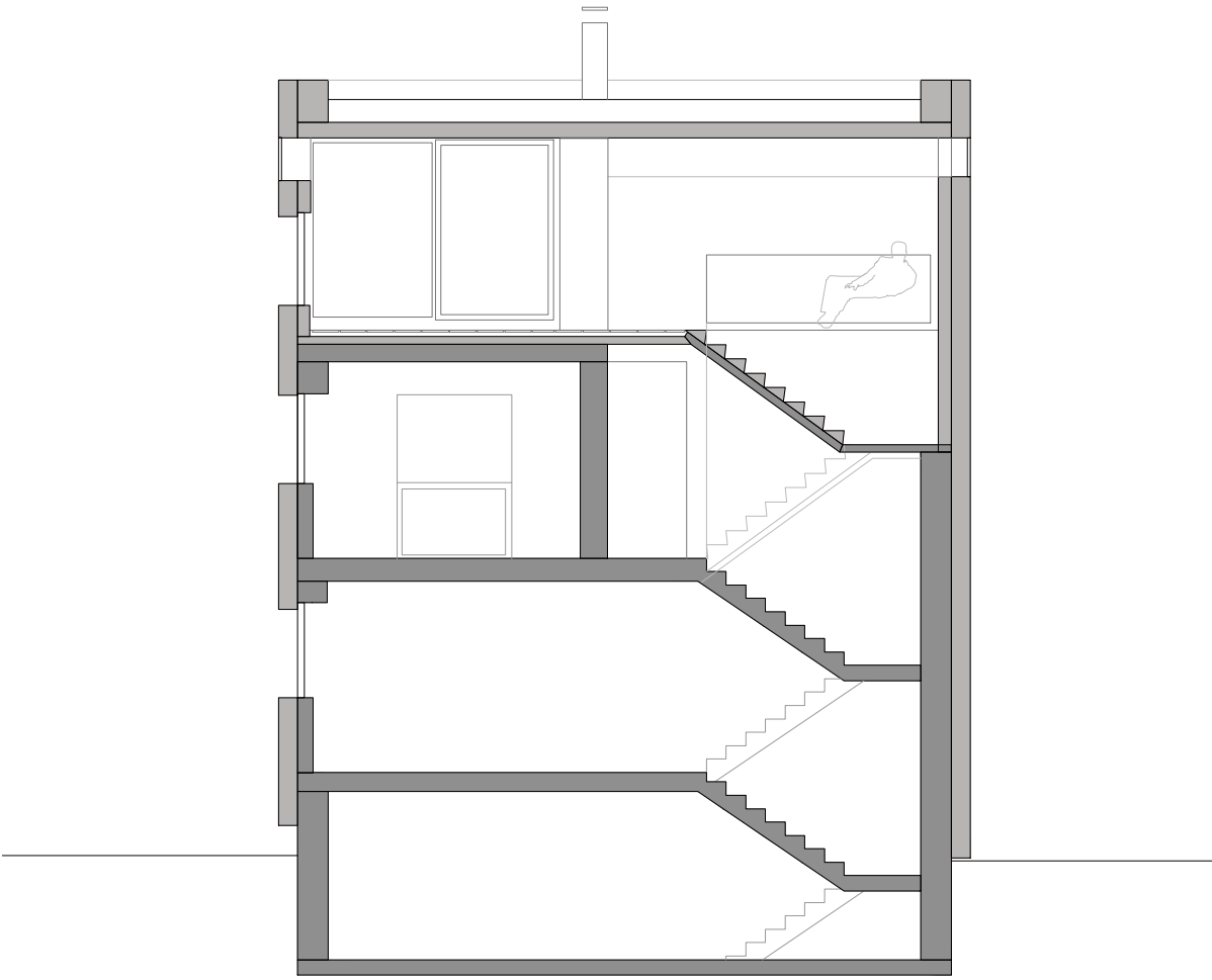
LÄNGSSCHNITT
