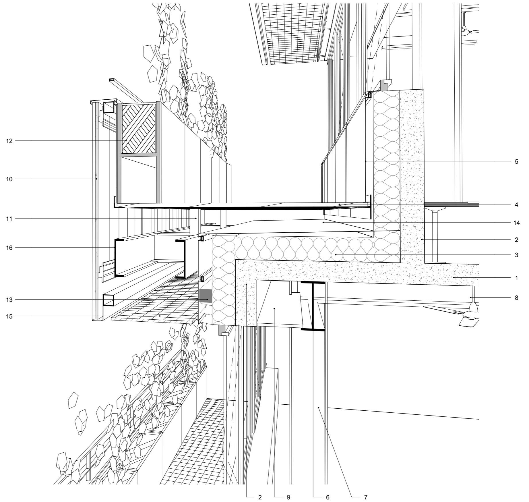
Détail 9 : Coupe coursière bavière/balcon - vue perspective
