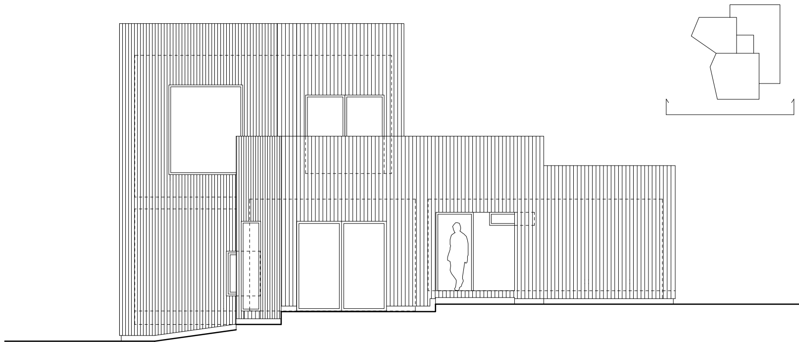
Facade/syd 1 : 50
