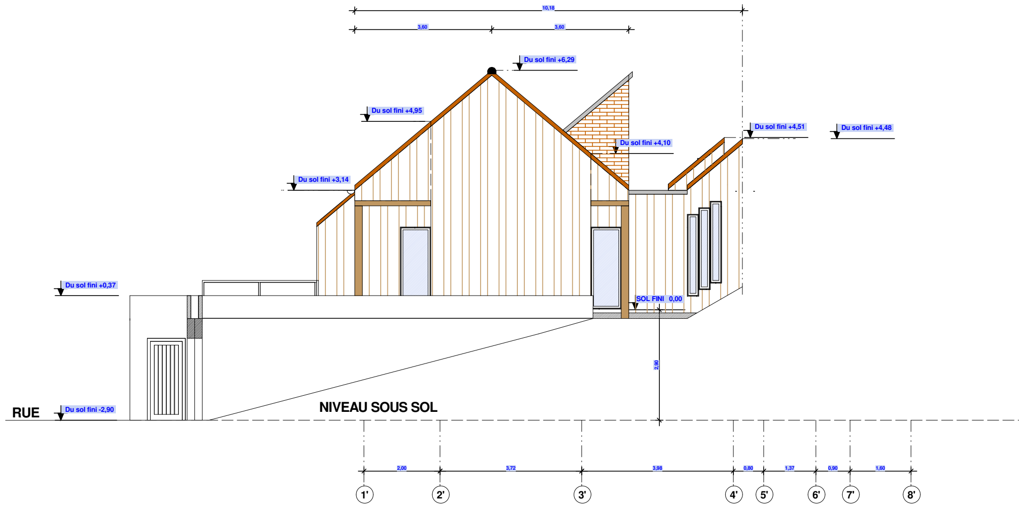
PIGNON OUEST
