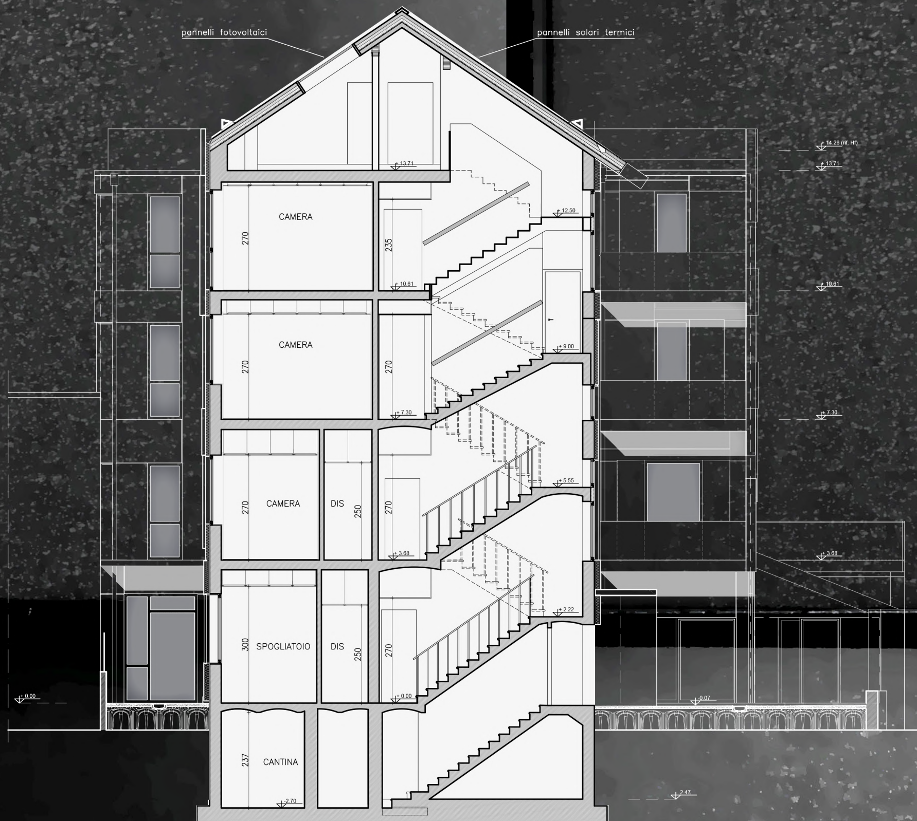
SEZIONE A - A FRONTE INTERNO SUD
