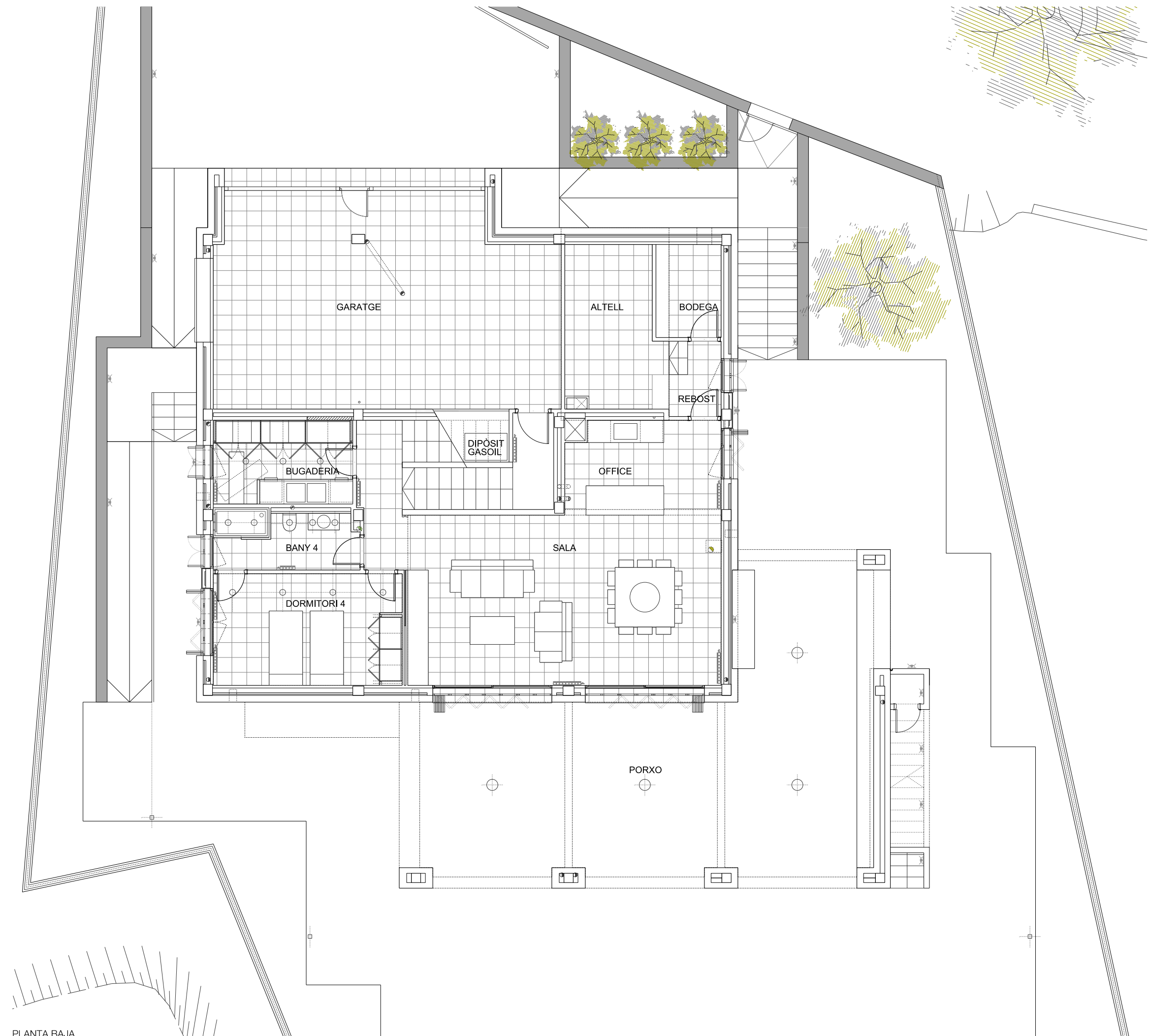
PLANTA BAJA
