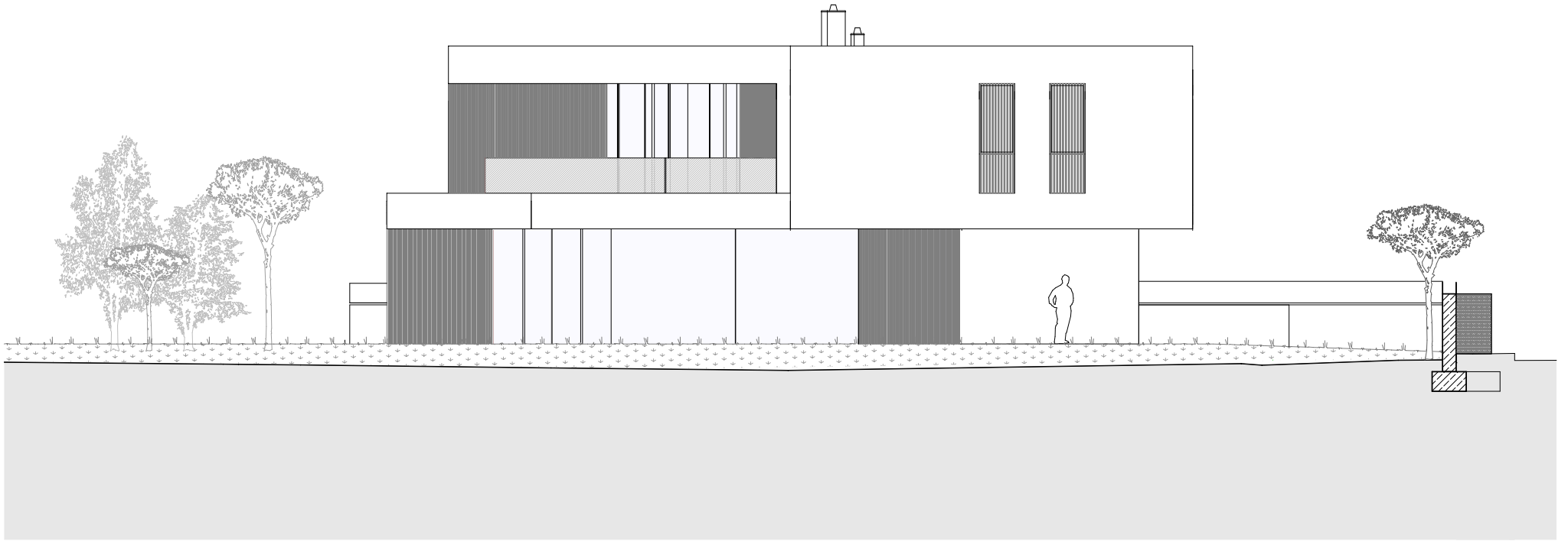
Ansicht Süd-Ost M 1:100
