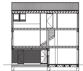
Langsdoorsnede
