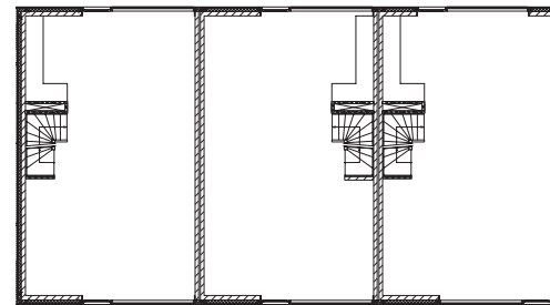
1e verdieping
