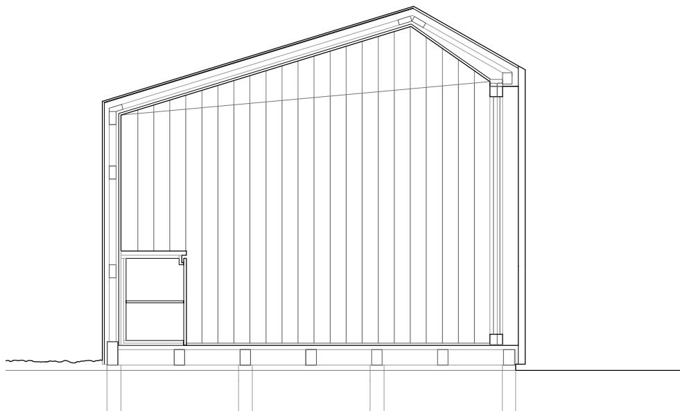
CORTE B
