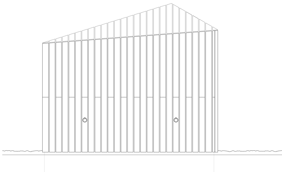
ALÇADO LATERAL
