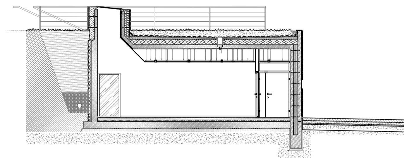
PRZEKRÓJ C-C
