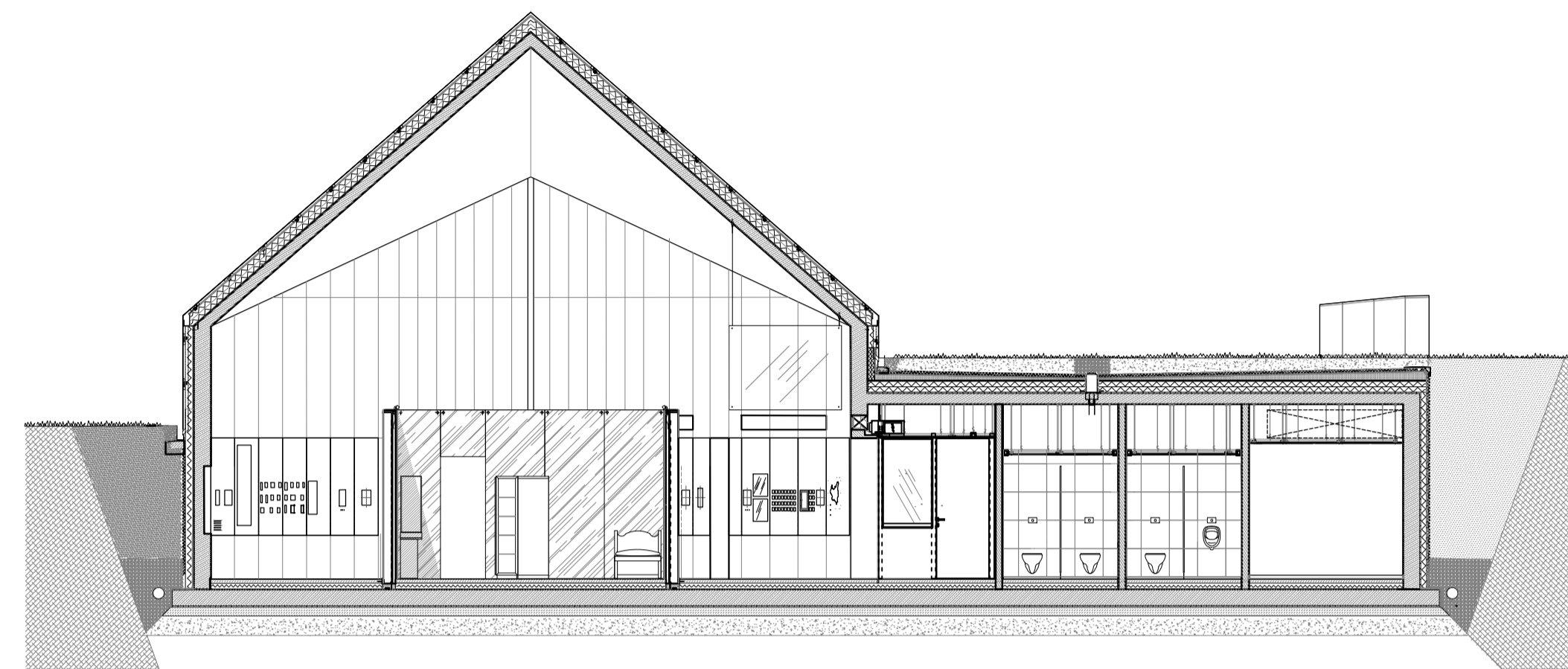
PRZEKRÓJ B-B
