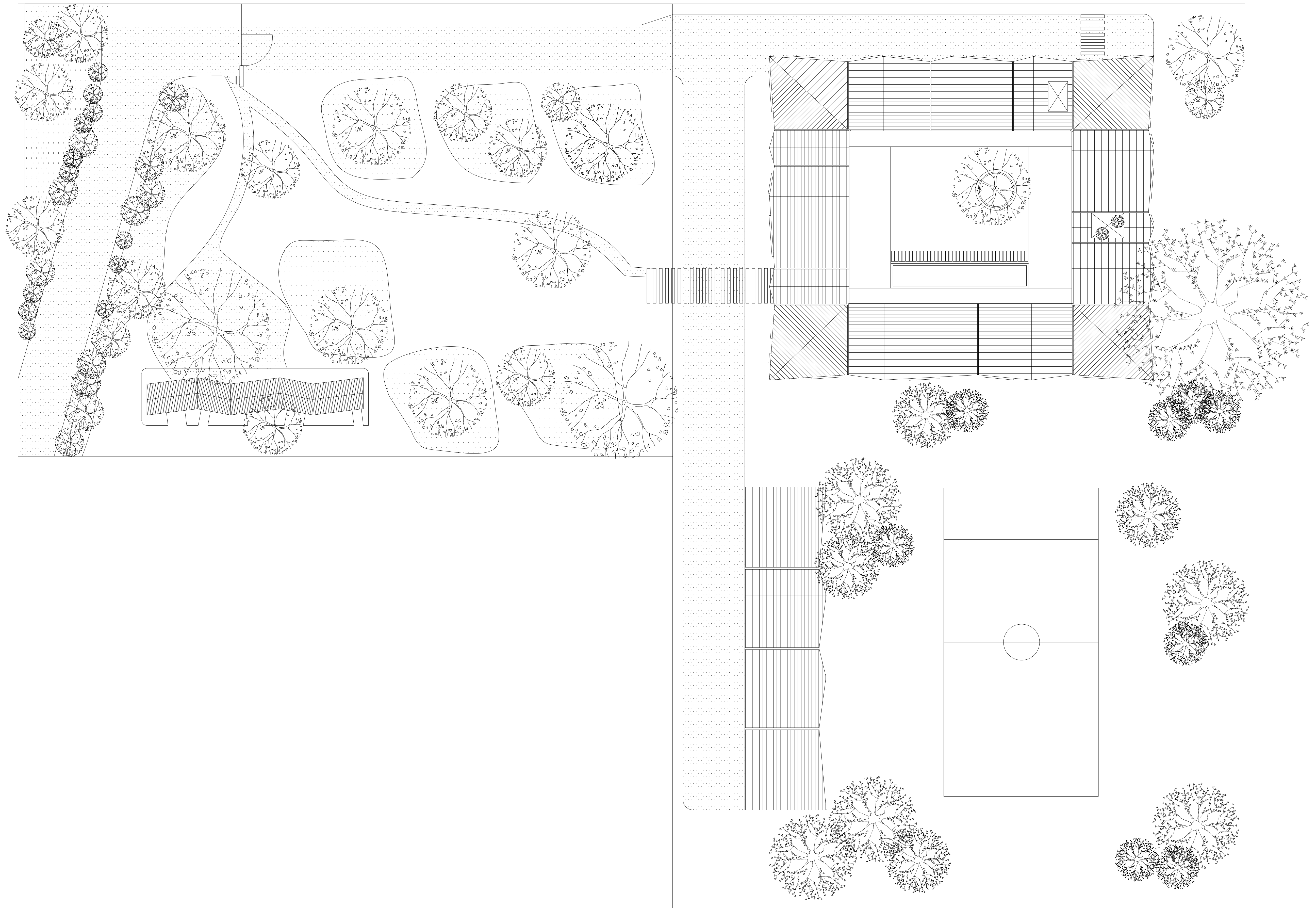
PLANTA EMPLAZAMIENTO
