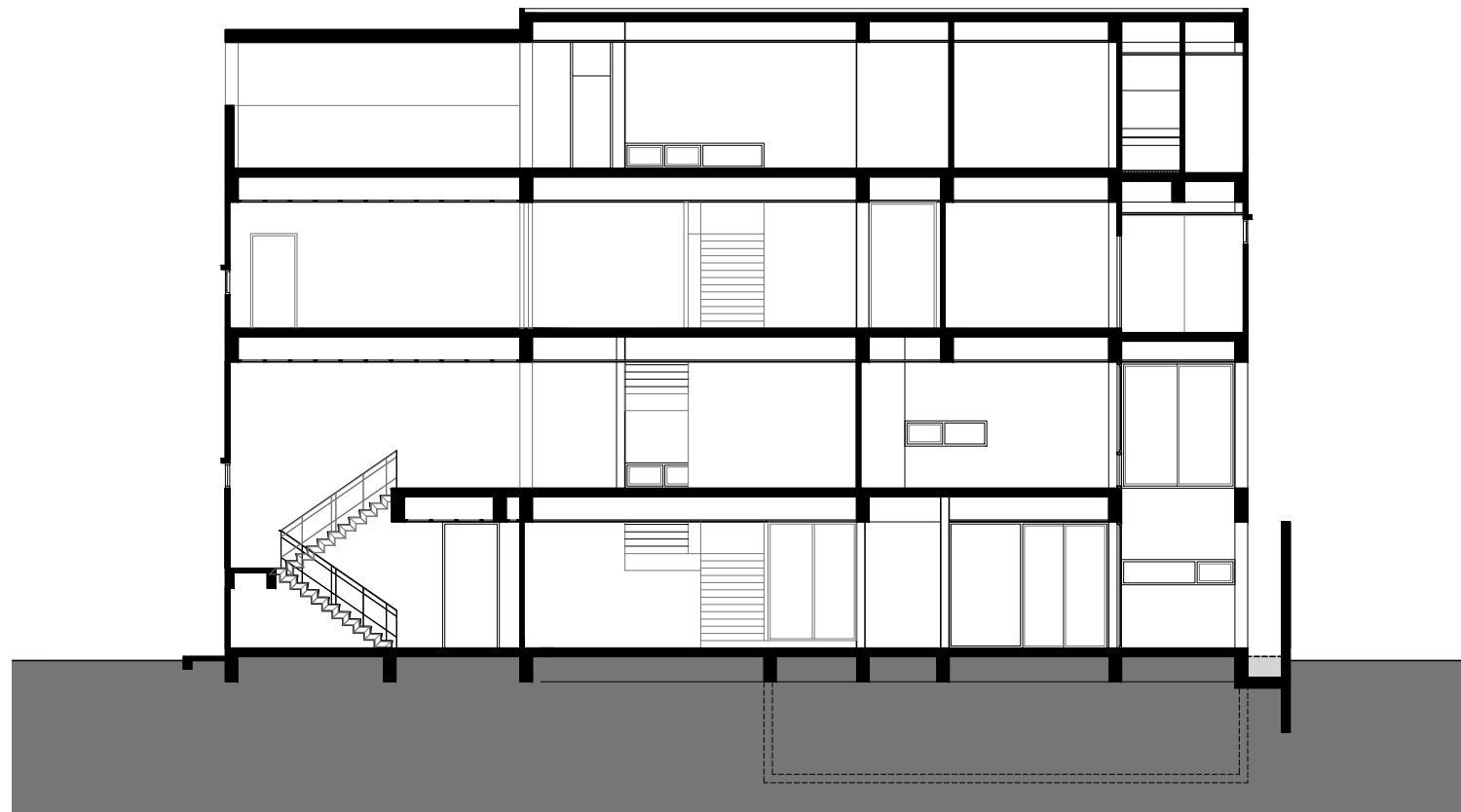
A-A SECTION
