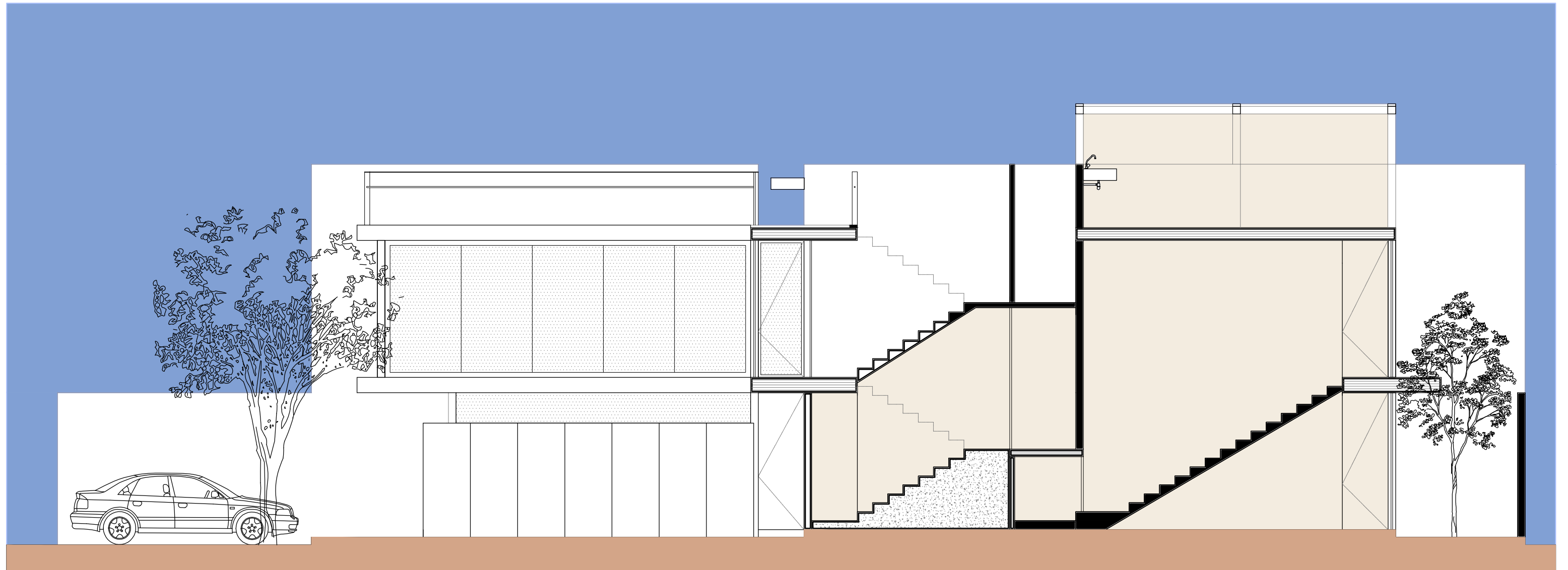
CORTE B-B'
