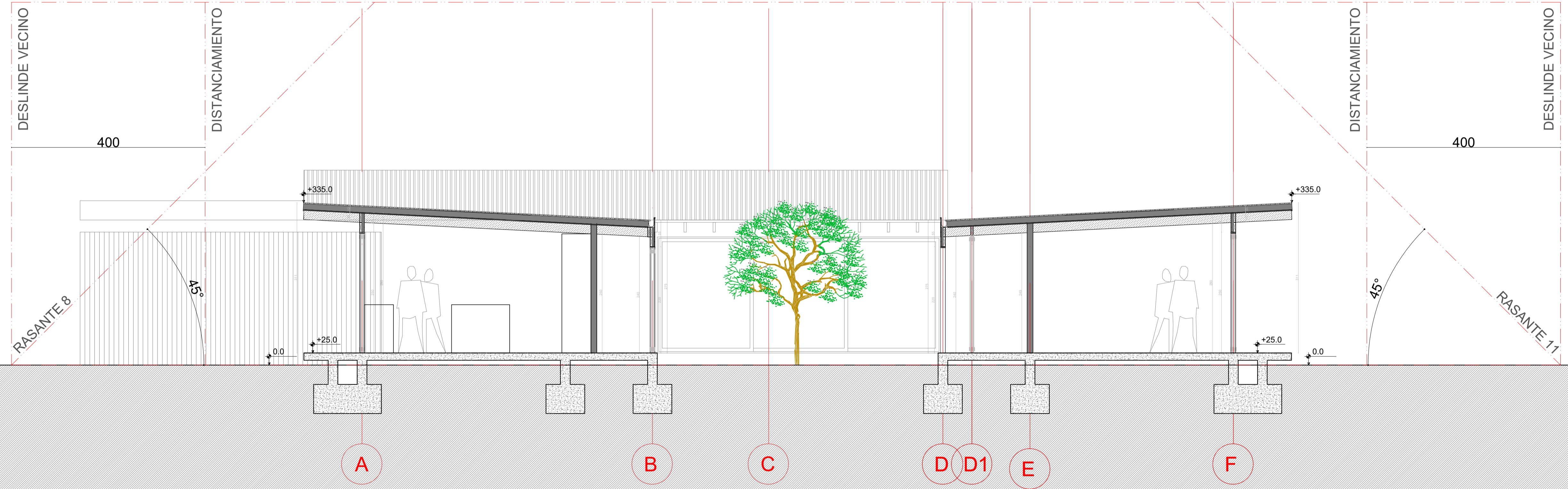
CORTE TRANSVERSAL B-B'
