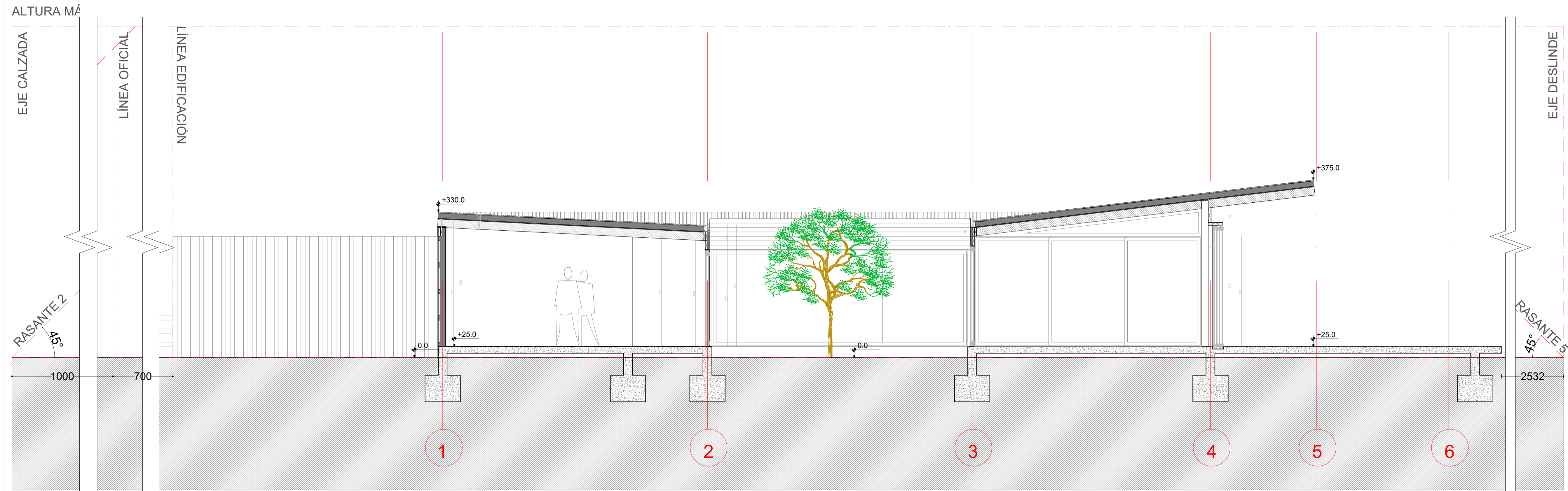
CORTE LONGITUDINAL A-A'
