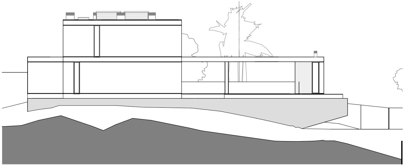
ALÇADO NORTE
