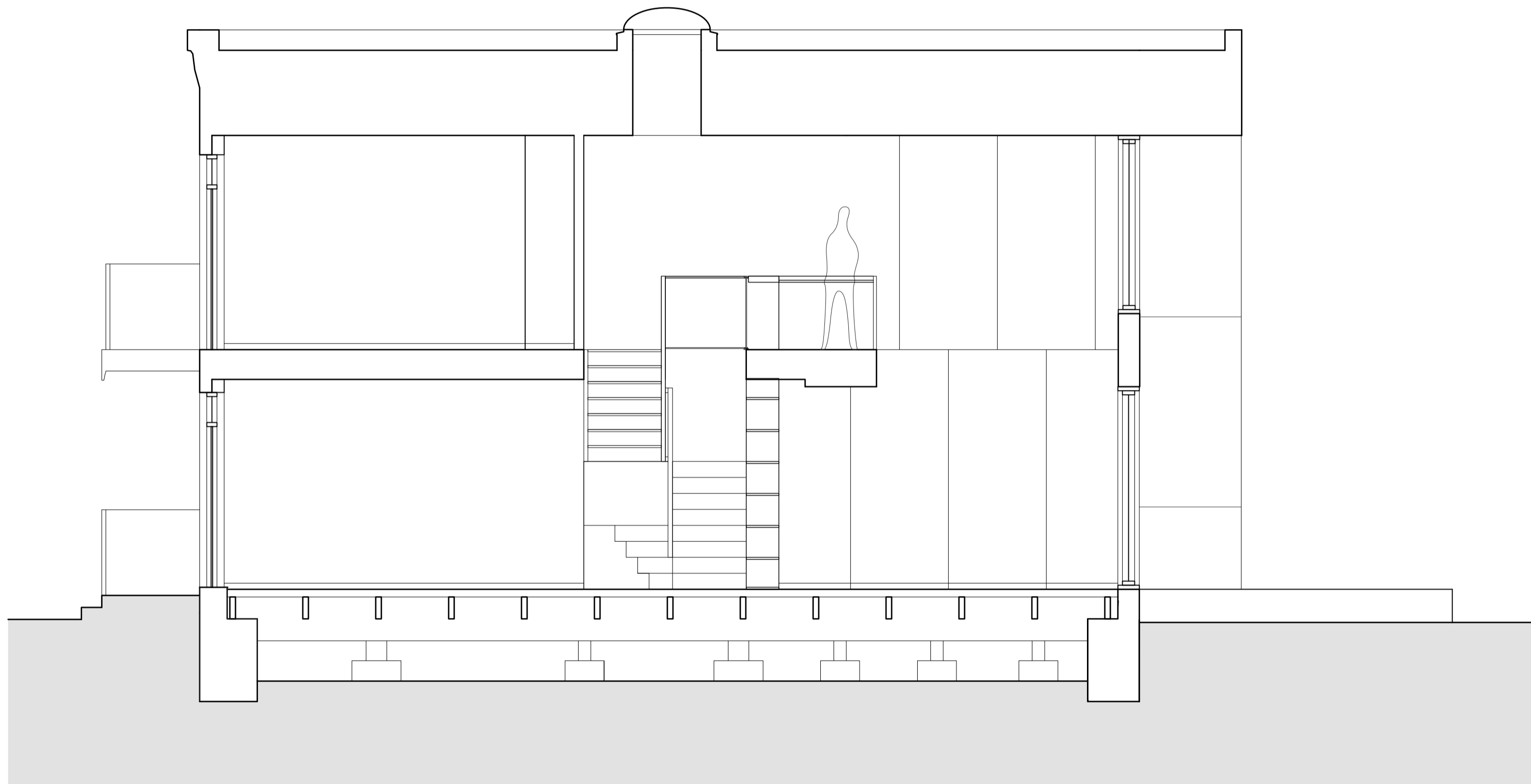
— COUPE LONGITUDINALE/ LONGITUDINAL SECTION
