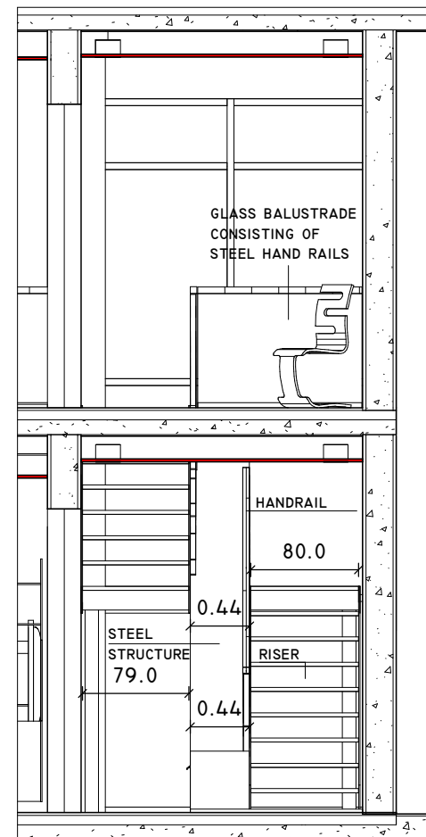
SECTION DD _ SCALE 1:50
