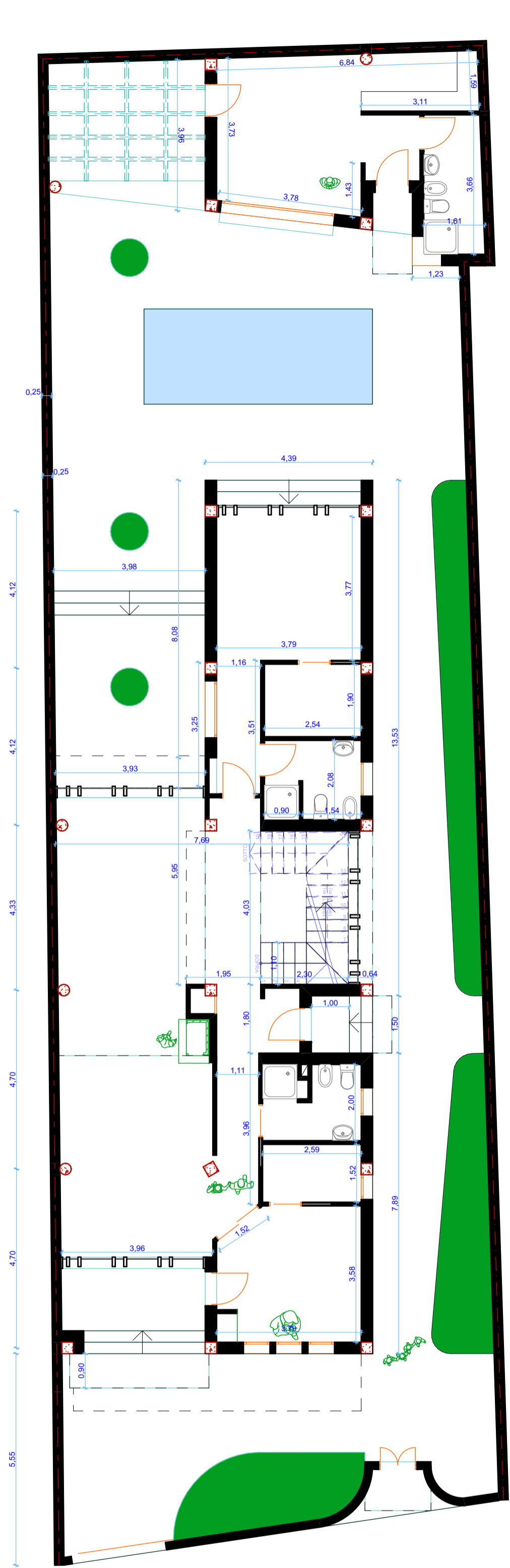
PIANTE QUOTATE
