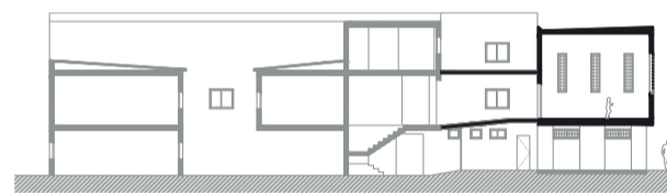
sección
