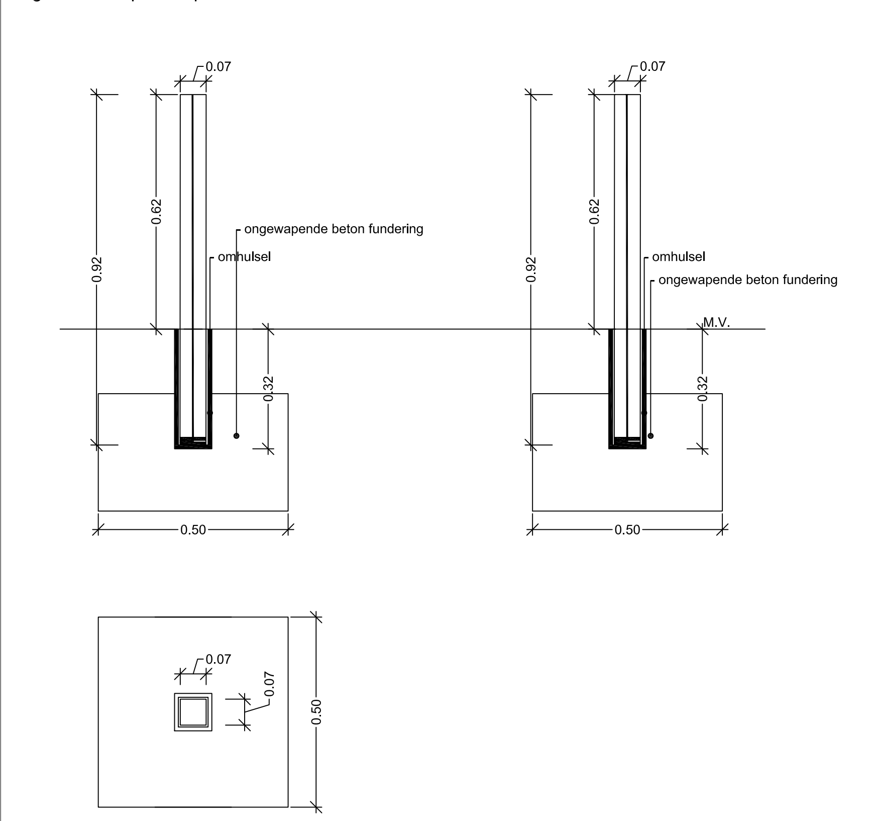
wegneembare parkeerpaal 1:10
