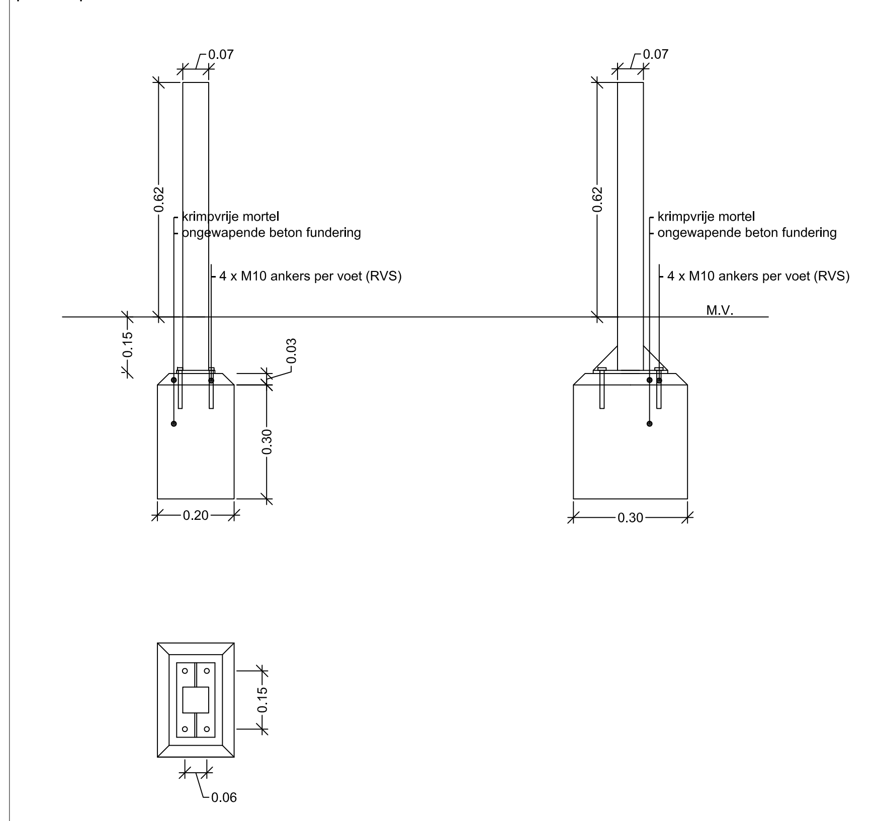
parkeerpaal 1:10
