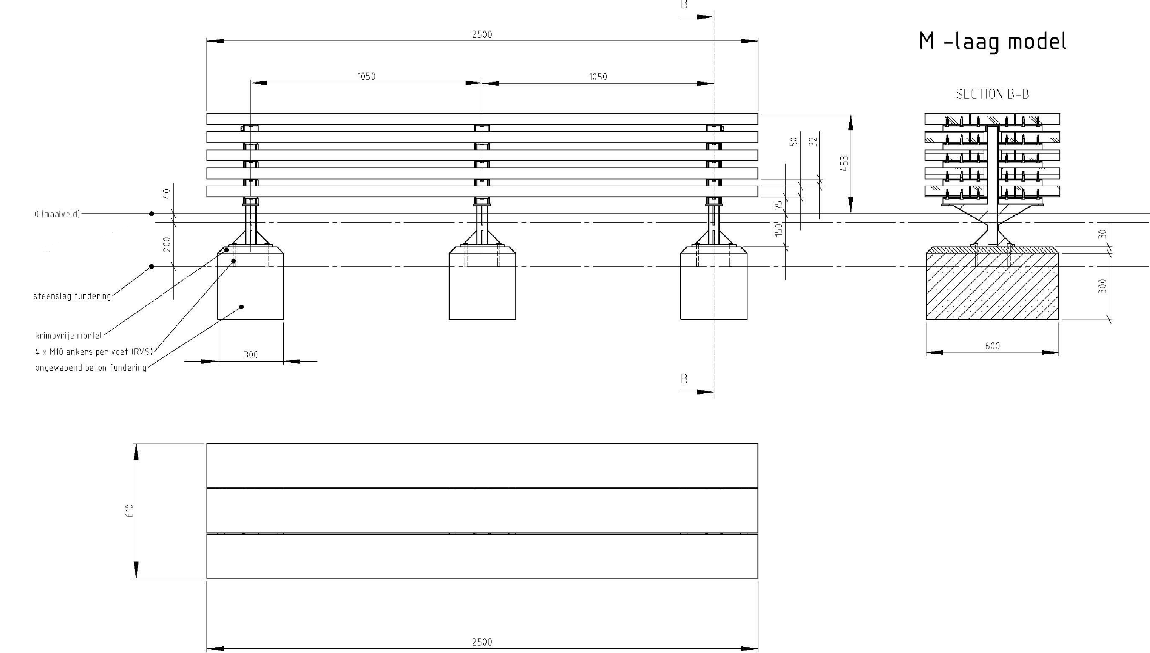
zitbank 1:10
