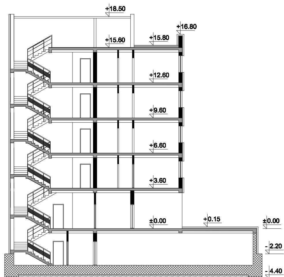
PRESEK B-B
