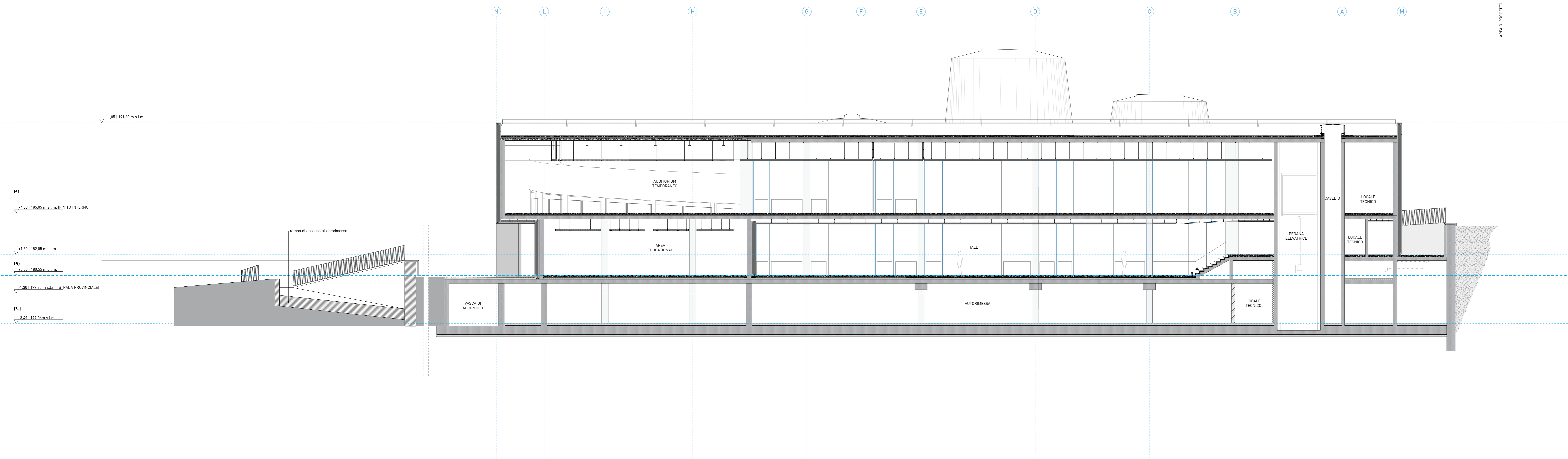
SEZIONE CC, scala 1:100
