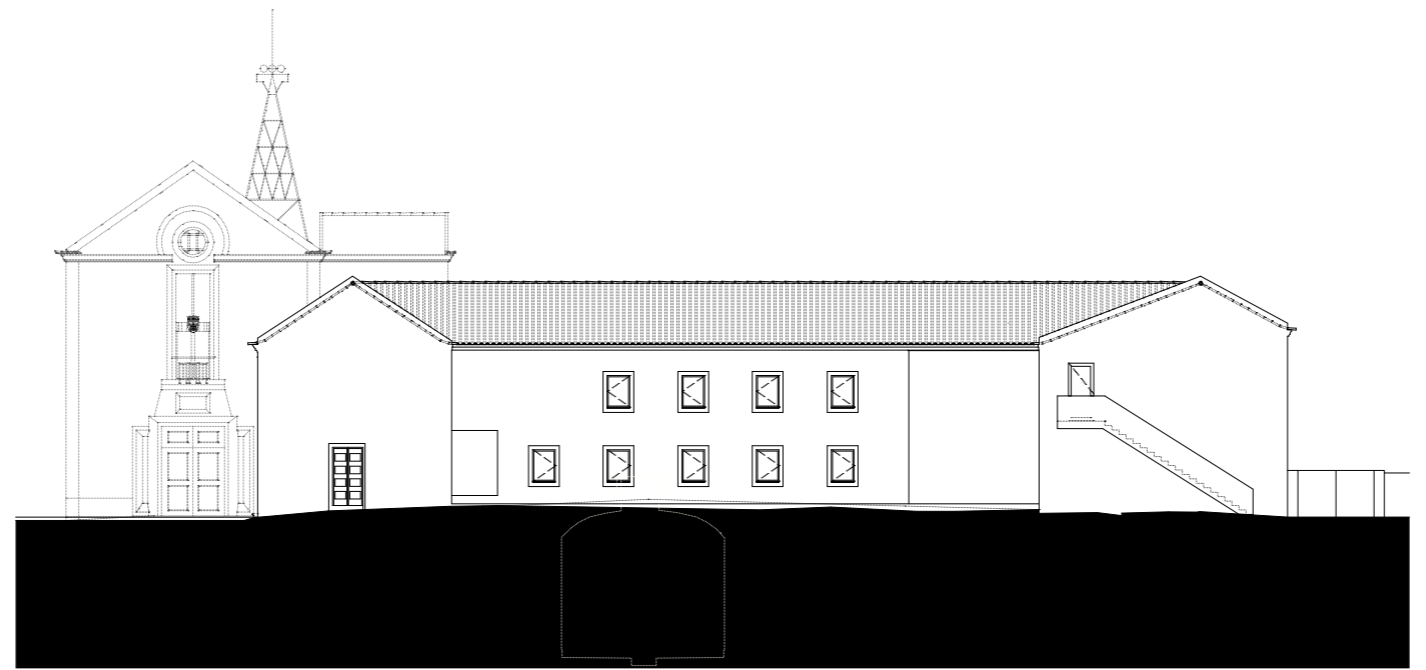
alçado poente. west elevation
