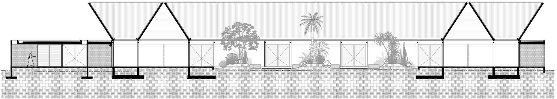
0 1 2 5 10 20 LONGITUDINAL SECTION CL2
