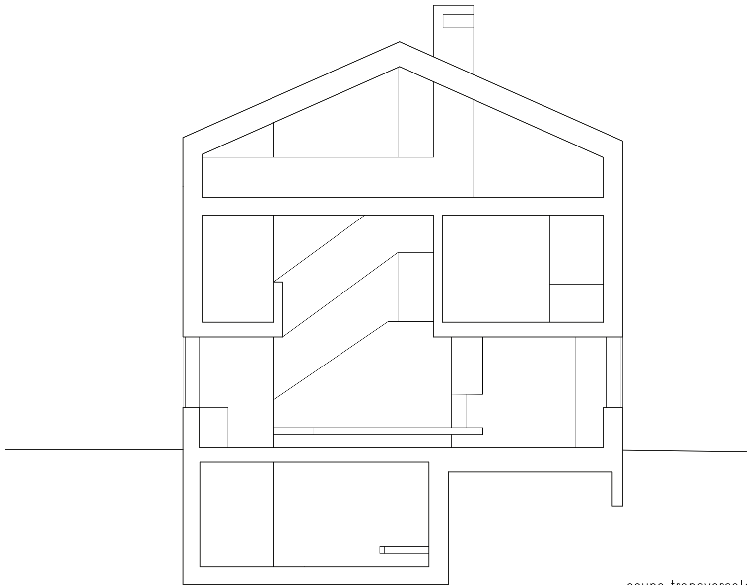
coupe transversale
