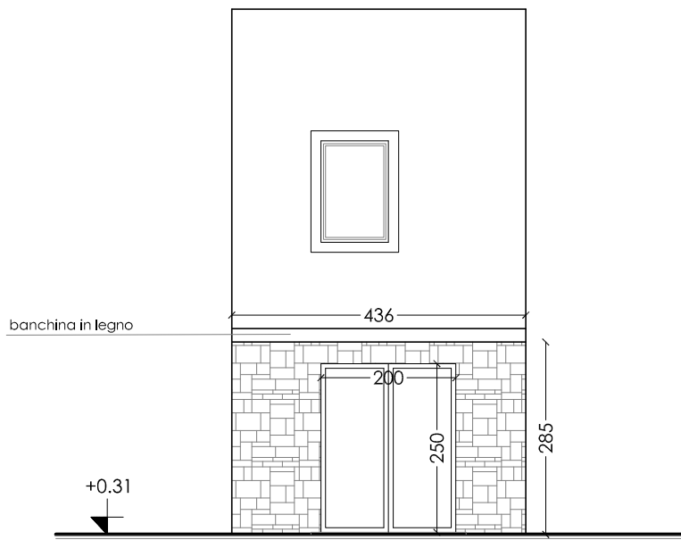
PROSPETTO SUD-OVEST
