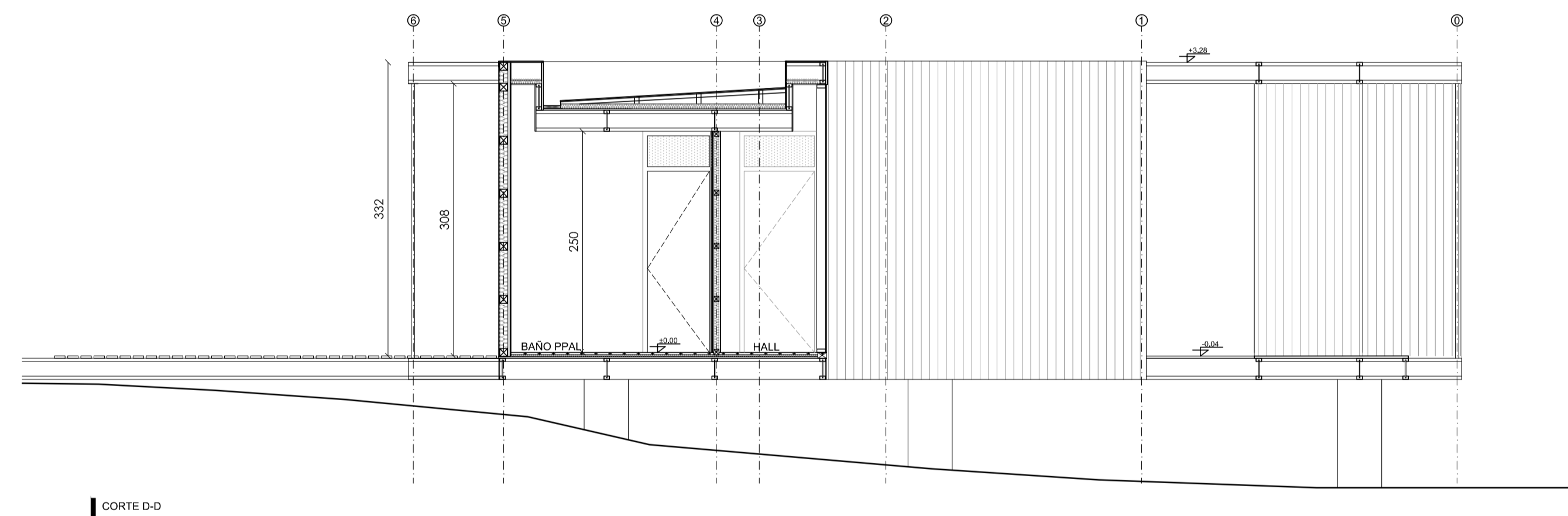
CORTE D-D
