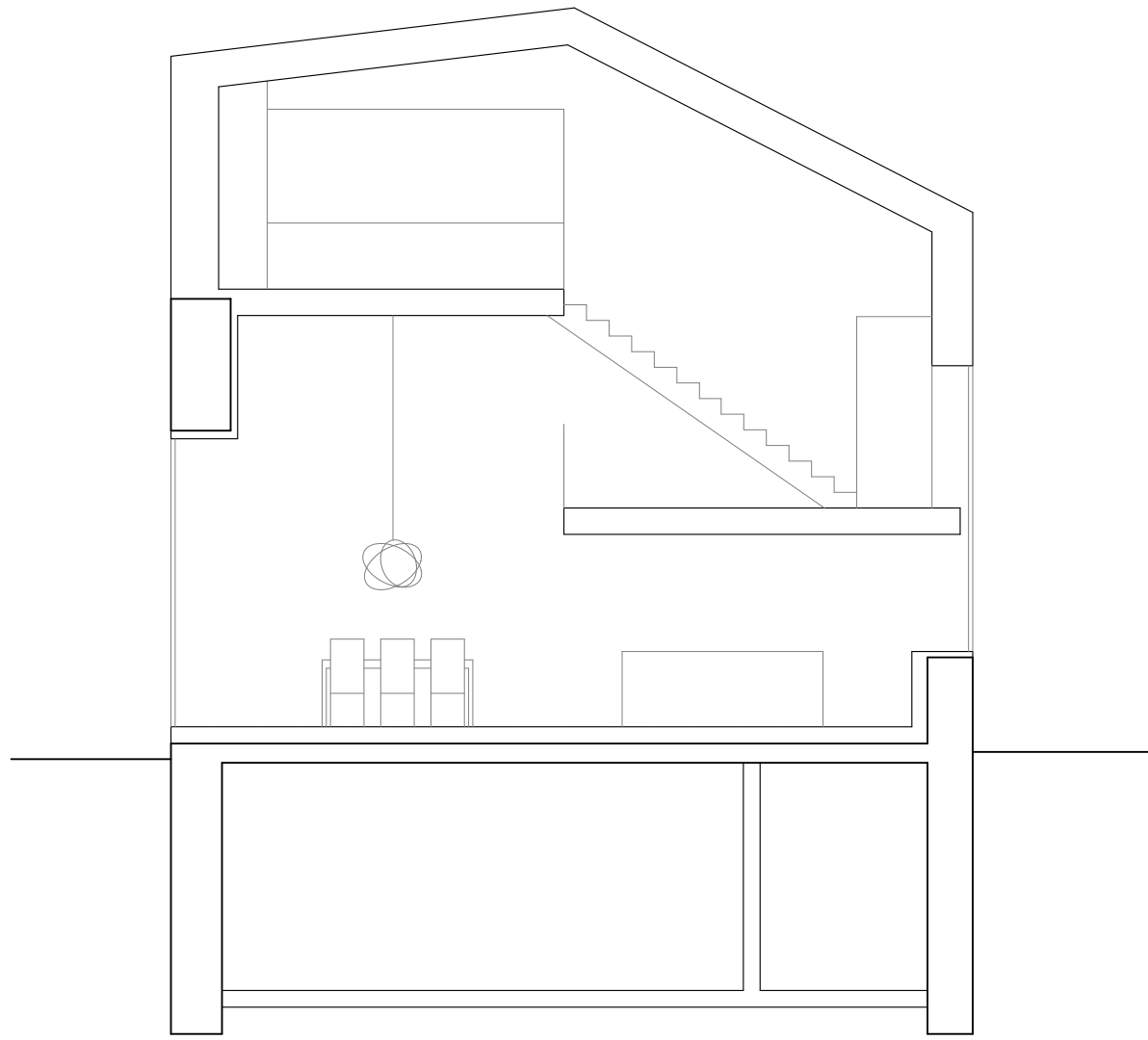
coupe transversale
