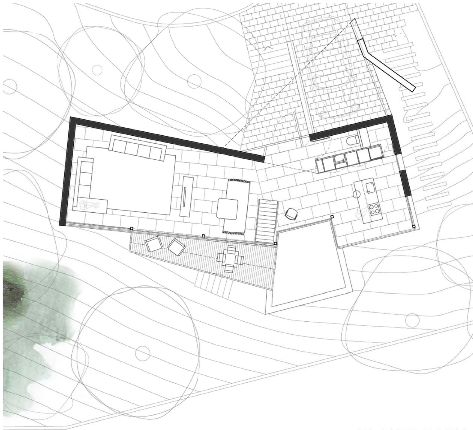
PLANTA BAIXA
