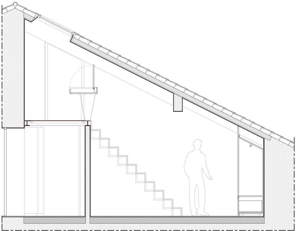
SEZIONE C-C'
